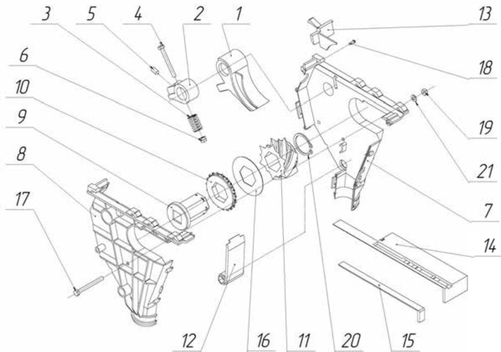
Рис. 3.6 Зерновой высевальной аппарат 400.00.3700А.
