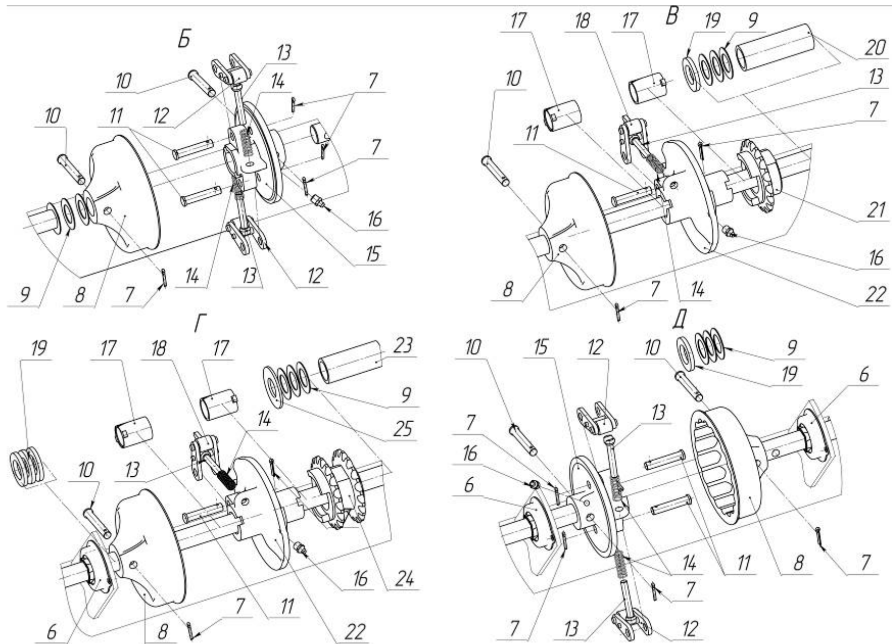
Рис.7.1.1 Валы контрпривода (продолжение).
