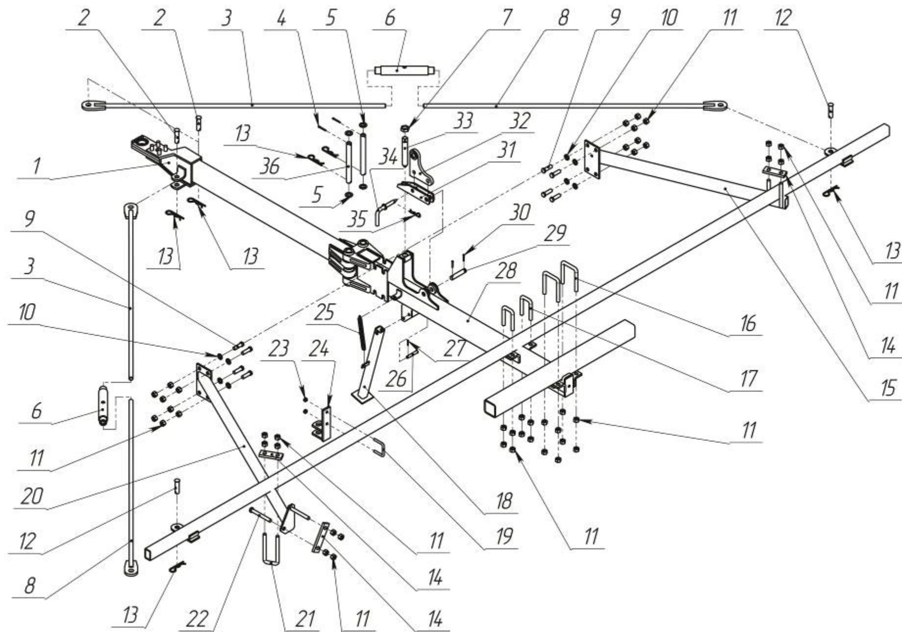
Рис. 17 Прицепное устройство.
