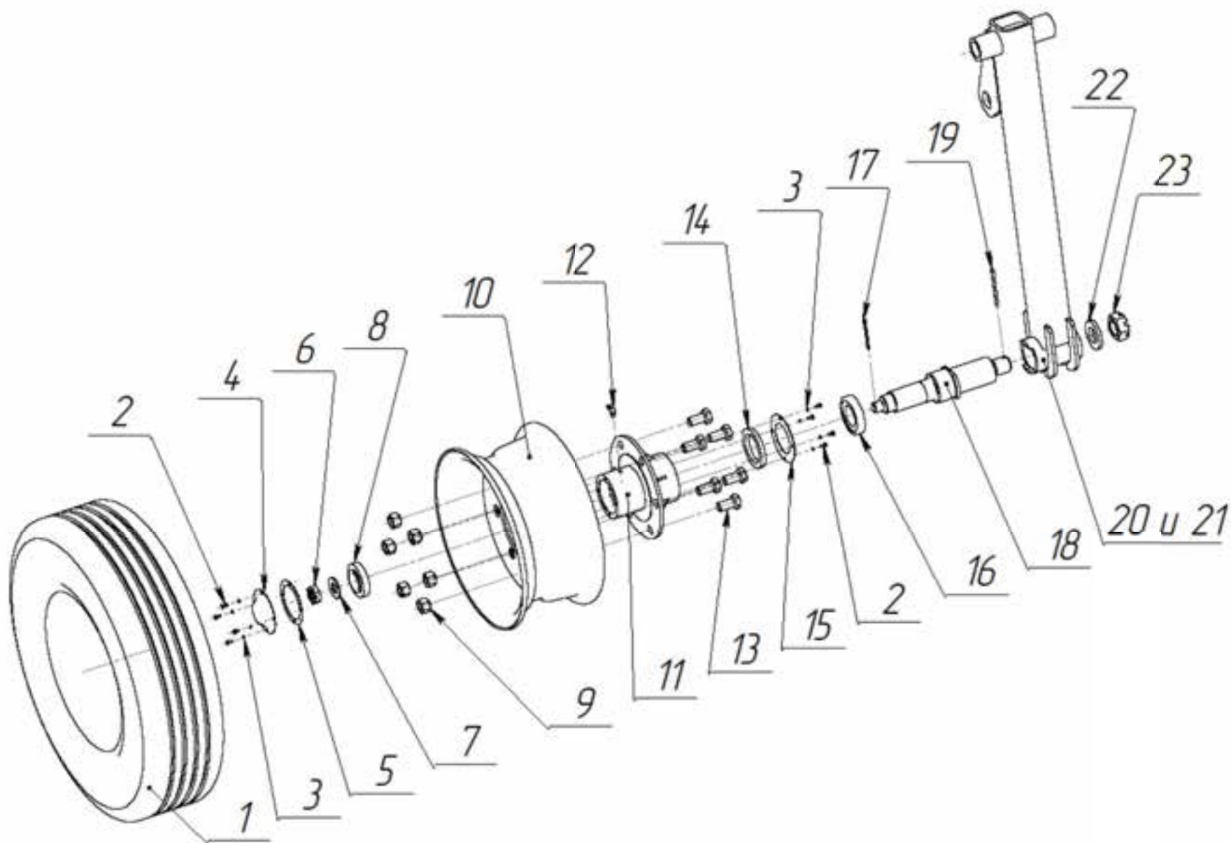
Рис. 5.1 Колесо ОЗШ 01.230.
