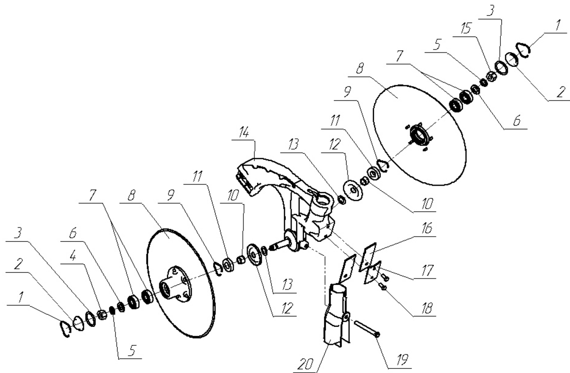
Рис. 12 Сошник Н 105.04.000.
