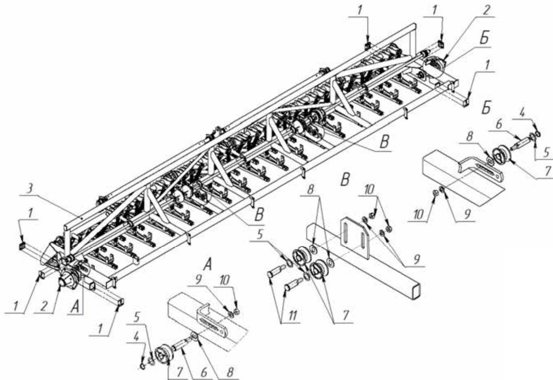
Рис. 7 Рама.
