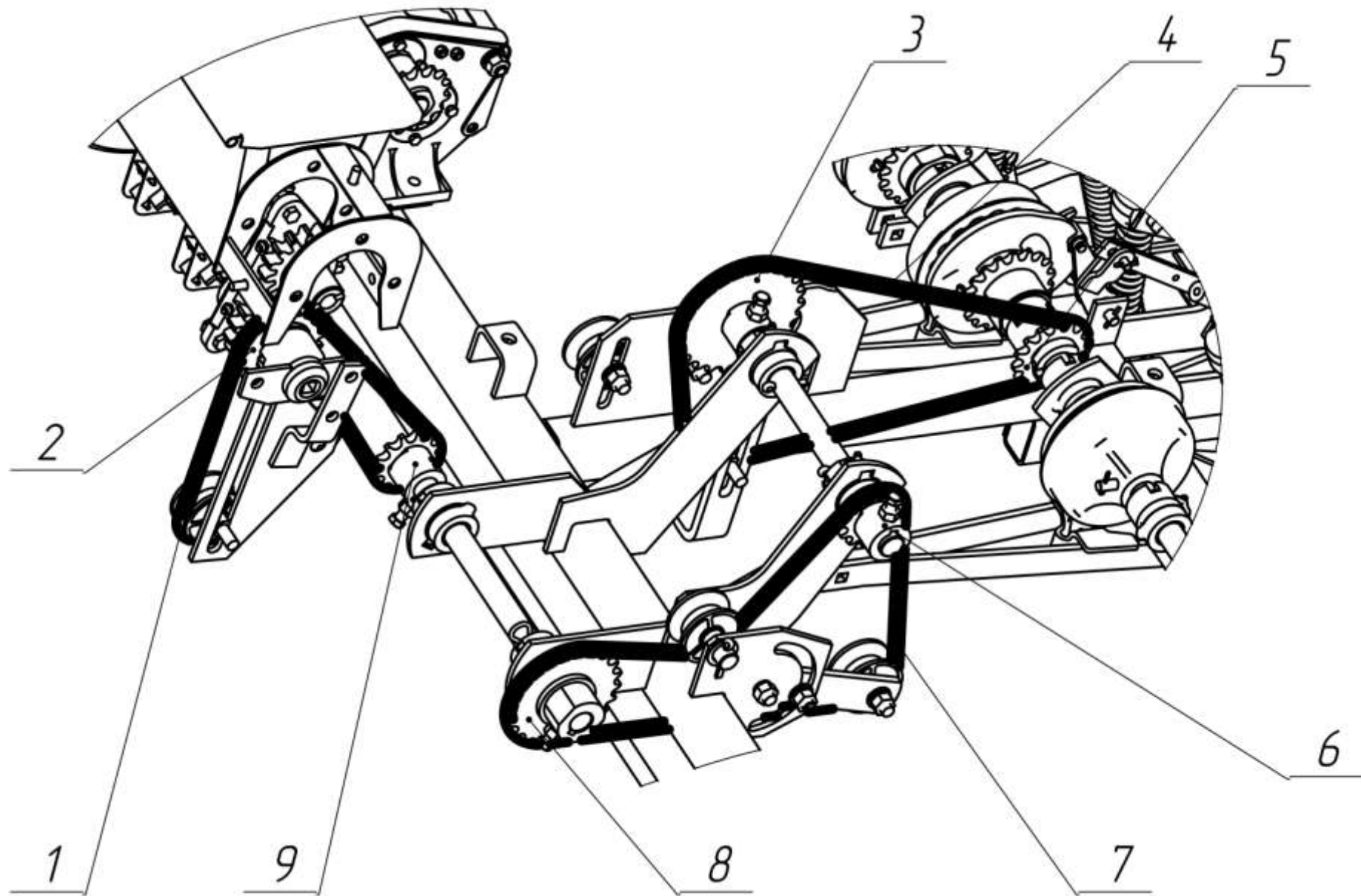
Рис.13. Механизм привода на валы травяных аппаратов
