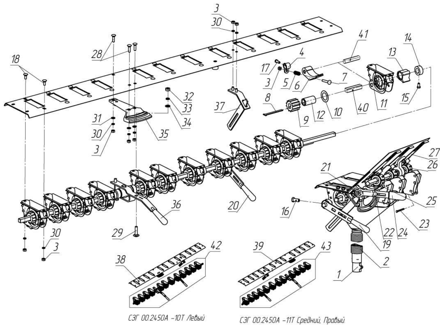
Рис. 6. Зерновой и туковый высевальные аппараты
