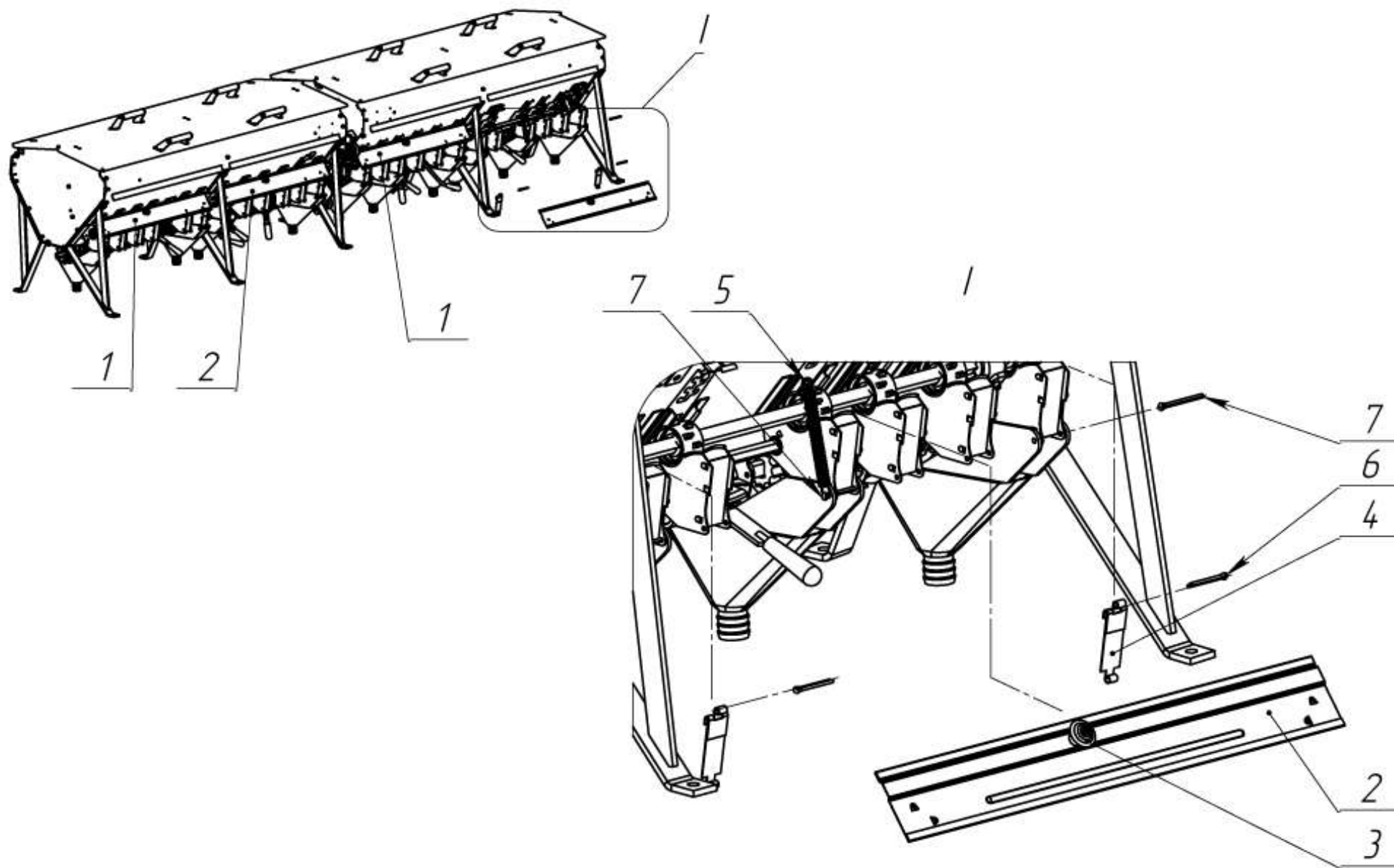
Рис. 5. Установка щитков туковывсевающих аппаратов
