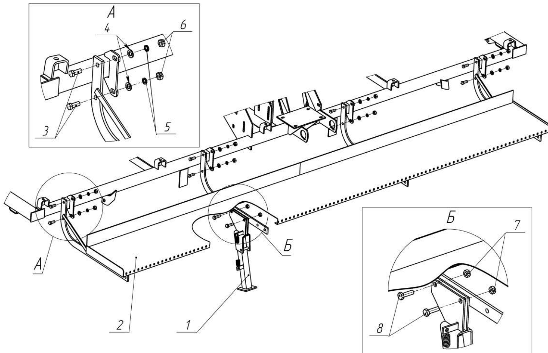
Рис. 25. Подножка ОЗШ 00.3010
