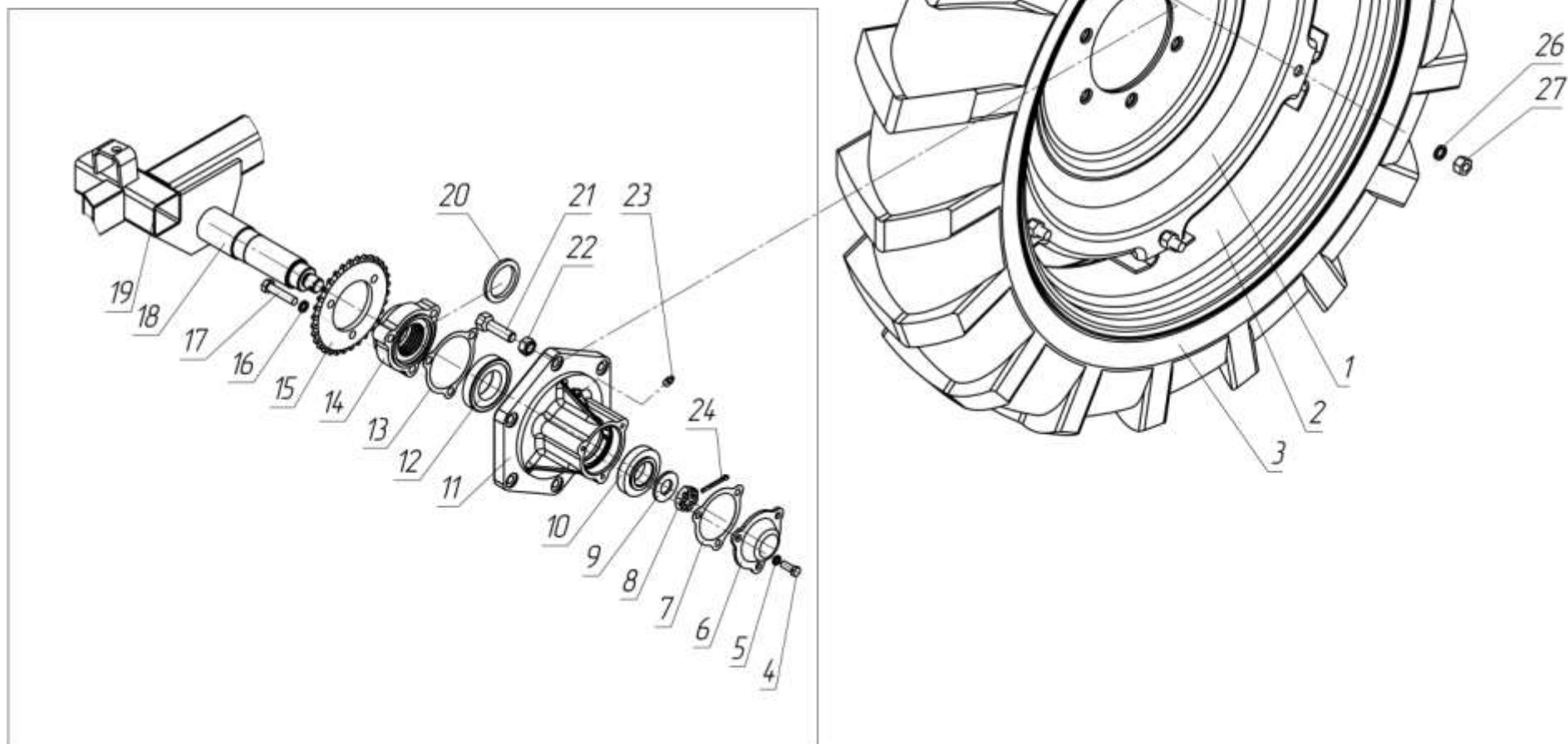
Рис. 3 Колесо опорно-приводное и ось СЗГ 00.1510 в сборе
