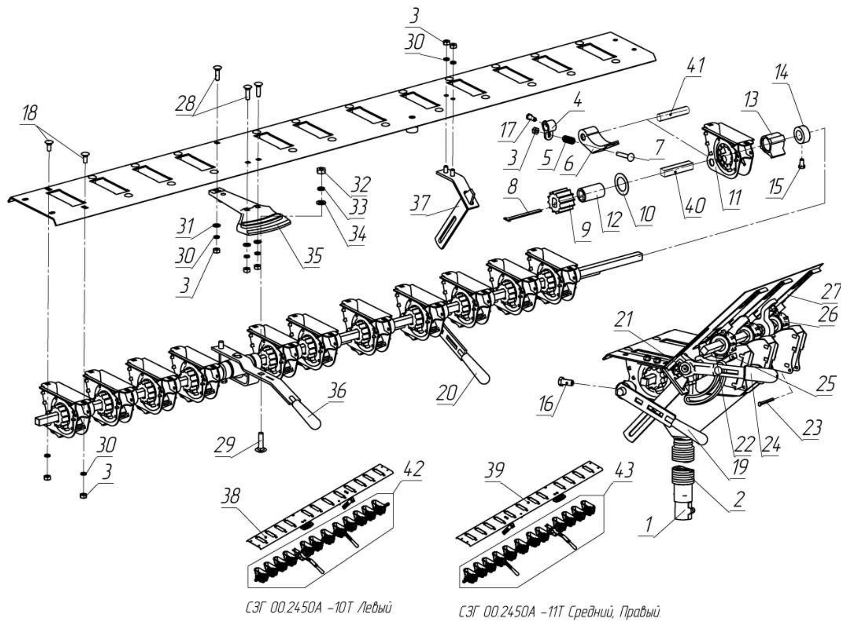
Рис. 6. Зерновой и туковый высевающие аппараты
