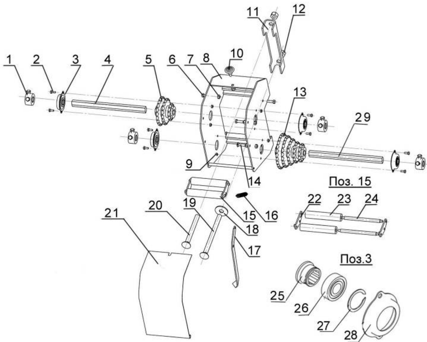
Рис.11 - Механизм передач СУС 00.180 (для «Веги-6»); СУС 00.180-01 (для «Веги-8»)
