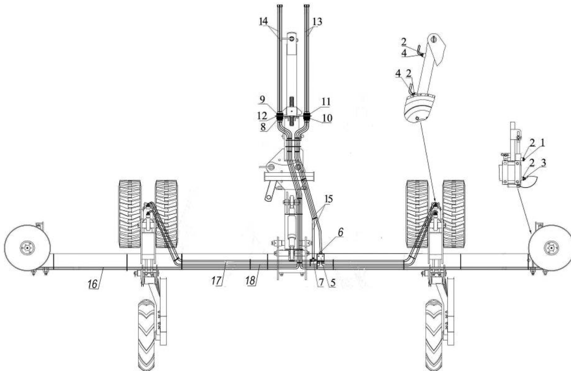
Рис. 25 - Гидротрасса управления маркером и опорными колесами СУС 00.5160
