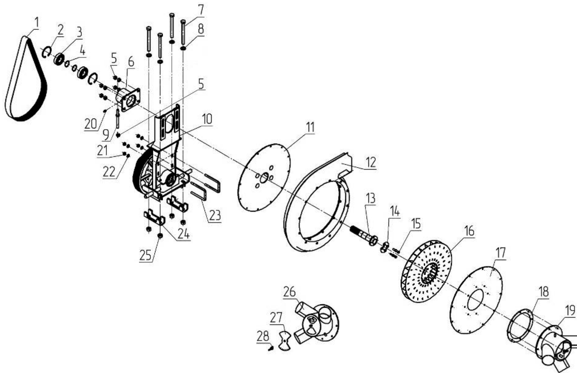
Рис.8 – Вентилятор 509.046.6150А-01
