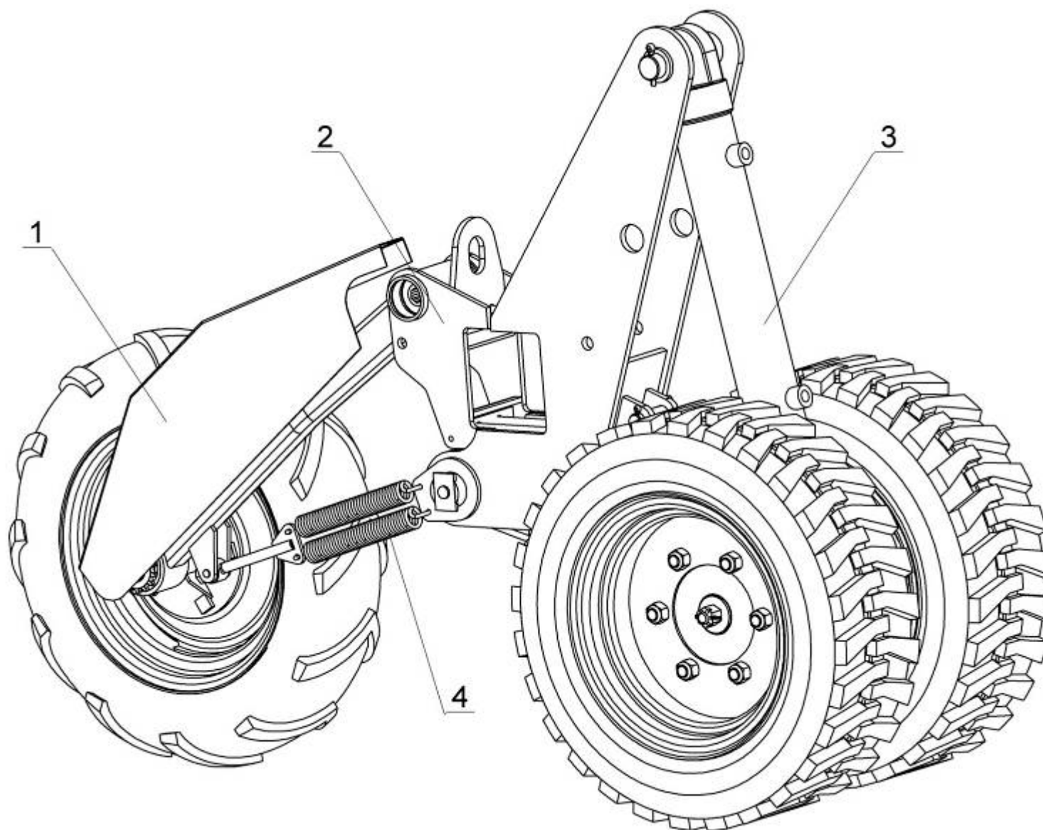
Рис. 12- Колесо опорно-приводное СУС 00.4970А
