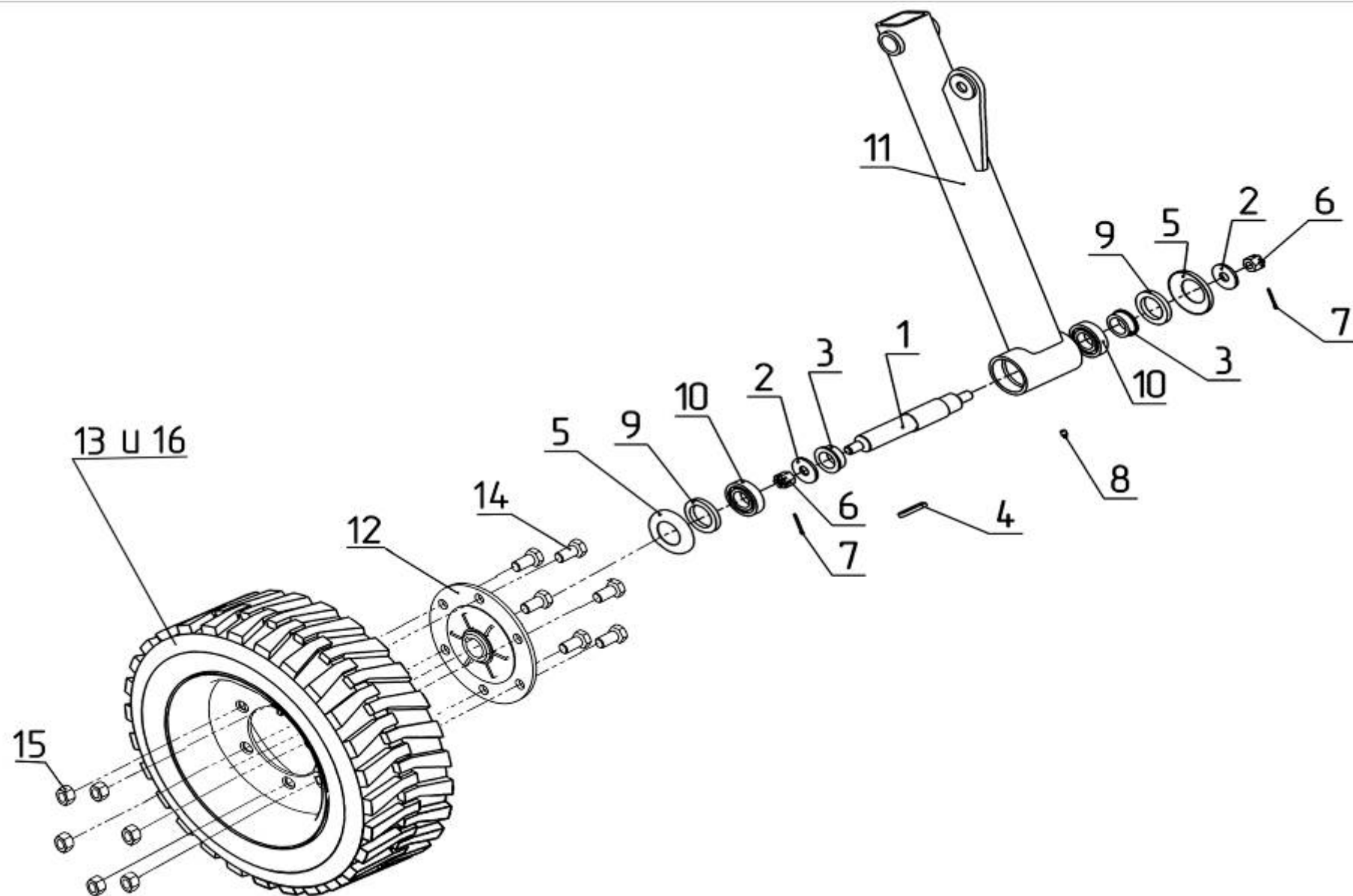
Рис.20 - Колесо СУС 00.2450 Колесо СУС 00.2450-01
