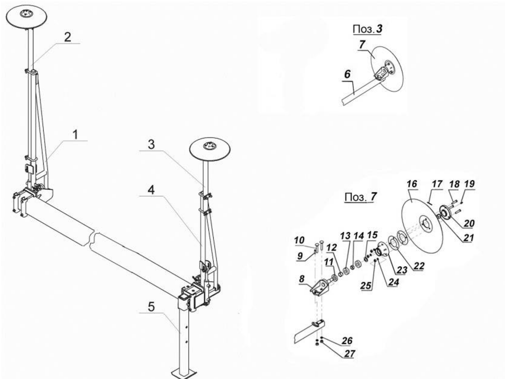
Рис.15- Маркер СУС 00.720А
