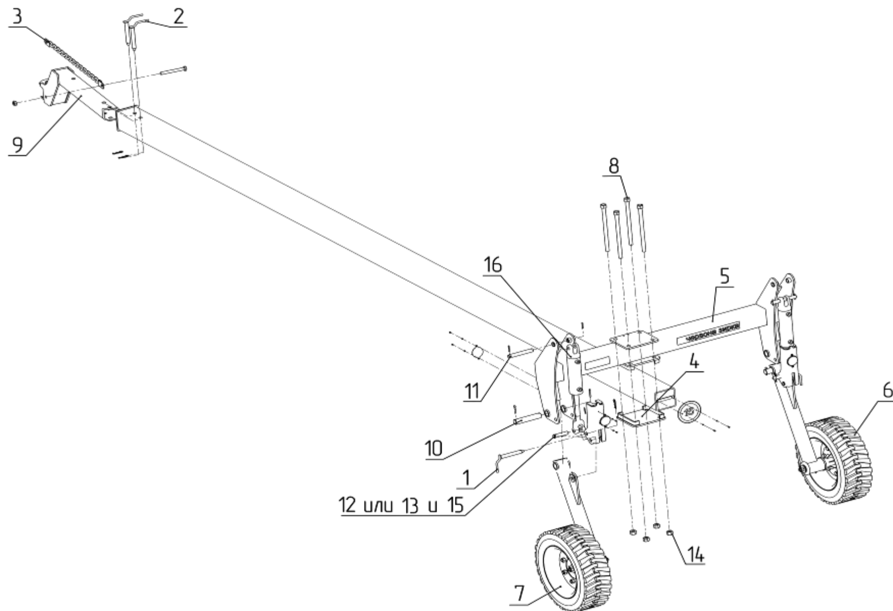
Рис.19 - Устройство транспортное СУС 00.1820А
