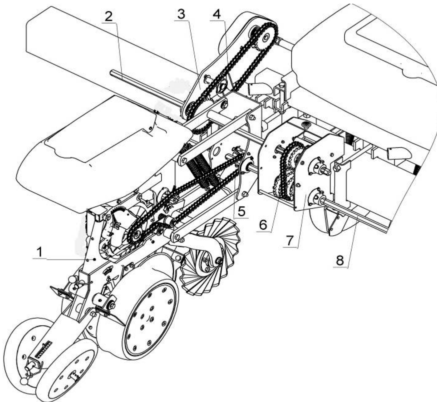
Рис. 24 – Привод посевной секции, редуктора и механизма передач.
