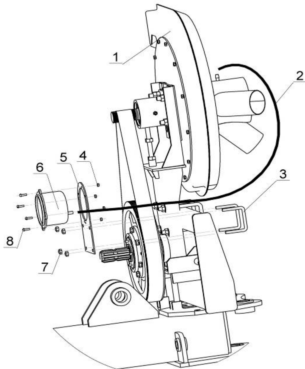
Рис.10- Подключение тягометра
