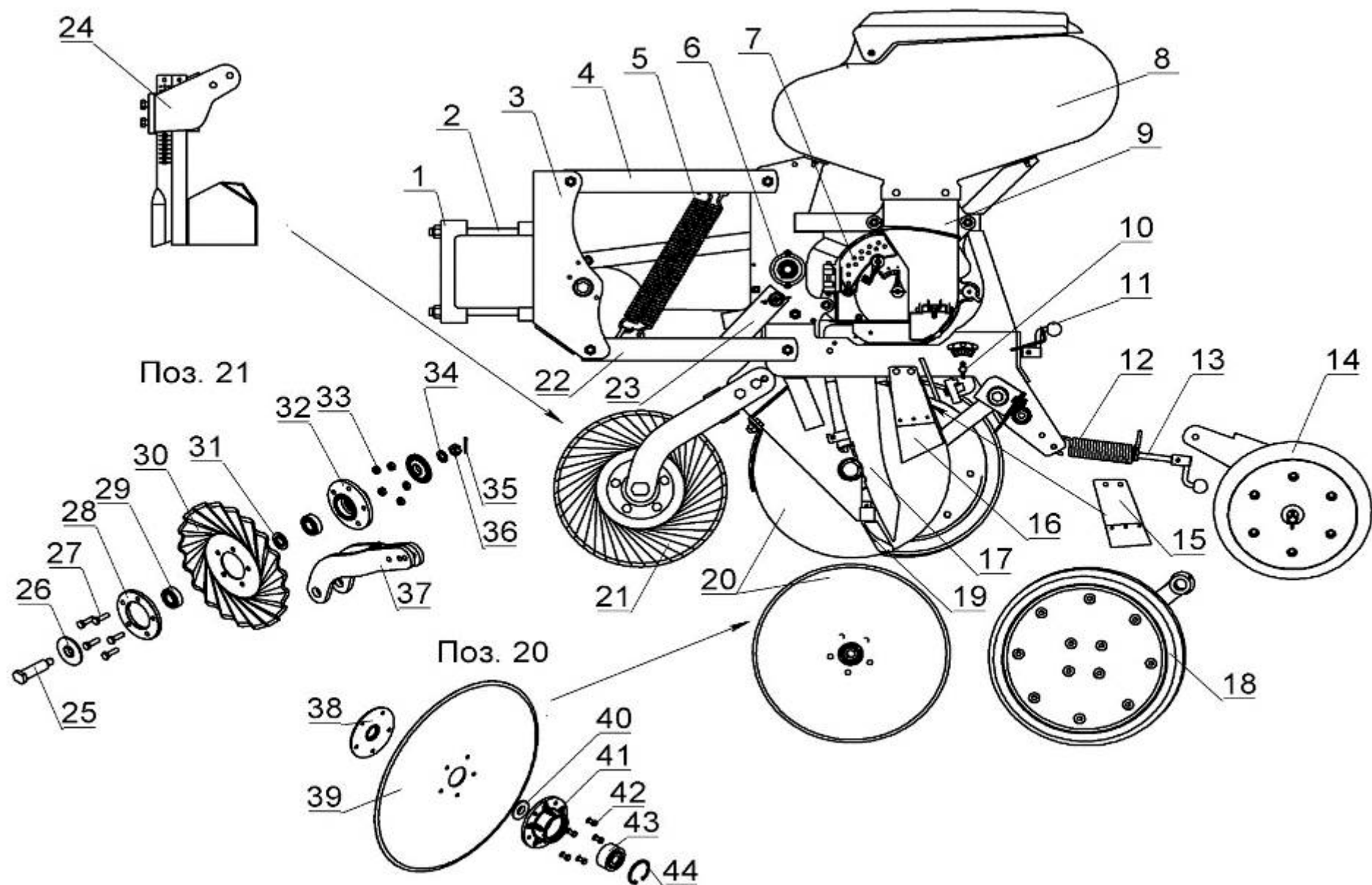
Рис.3 – Секция СУС 00.1600
