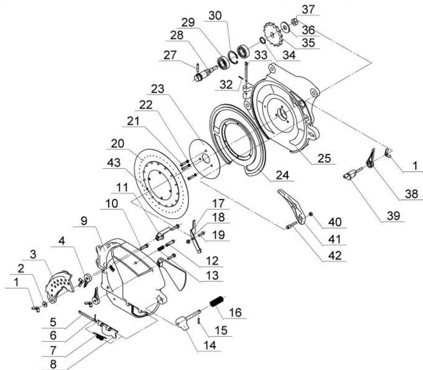
Рис.5- Аппарат высевающий СУС 00.1400-01
