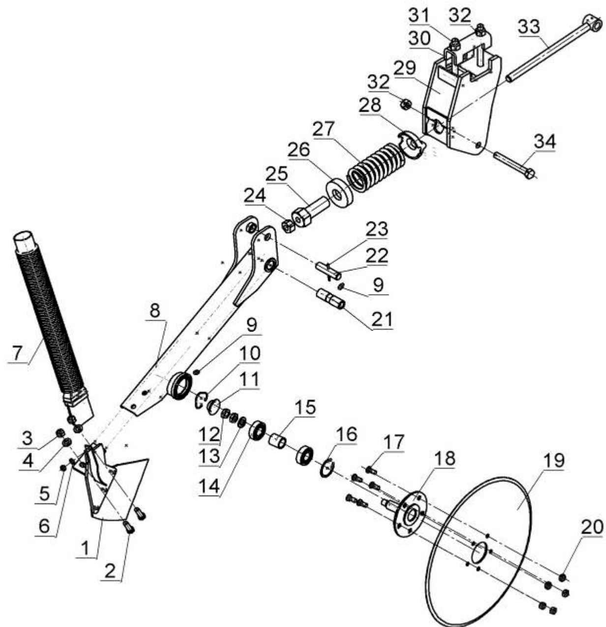
Рис.18 - Сошник туковый СУС 00.4600 (правый), СУС 00.4600-01(левый).
