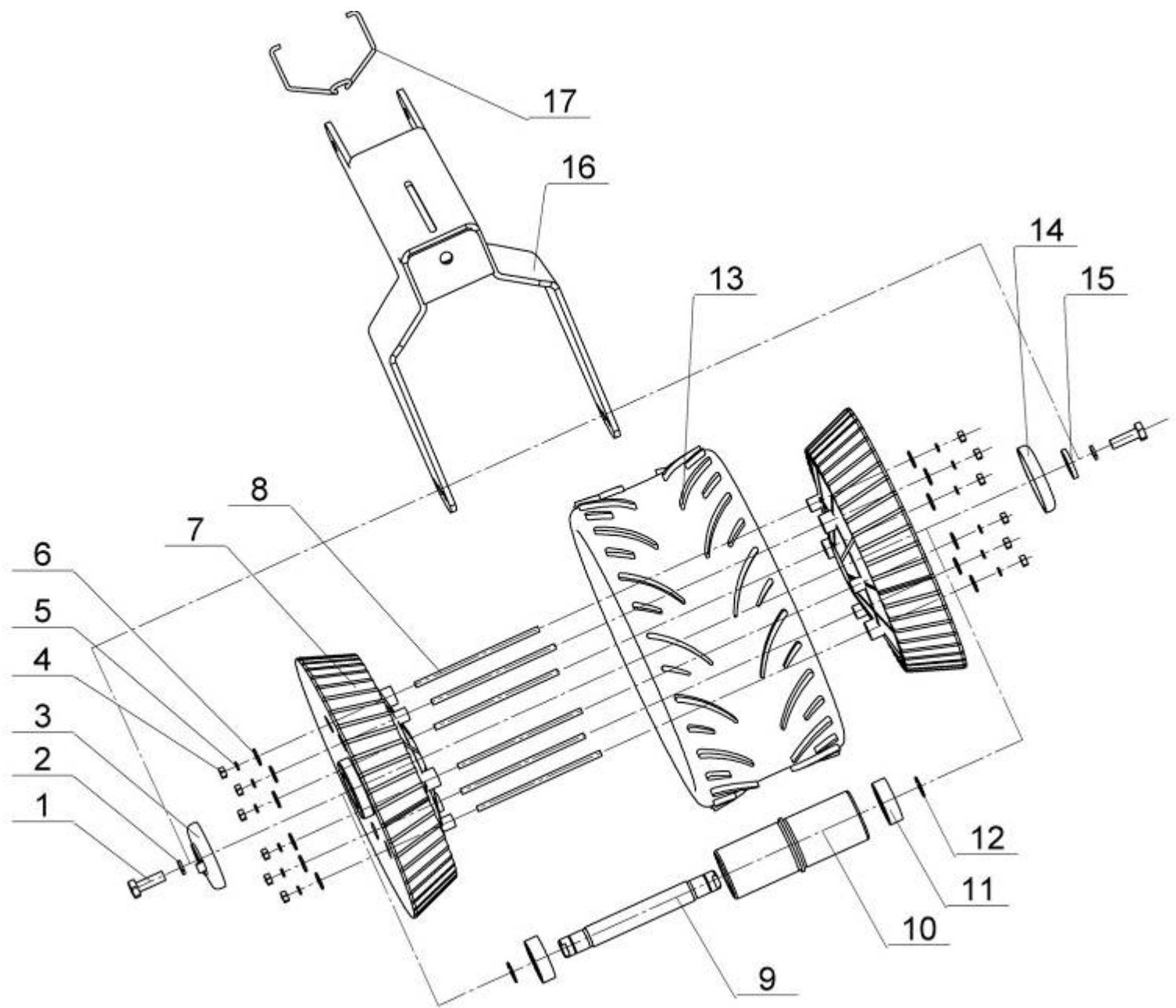
Рис.7 - Каток копирующий СУС 00.130
