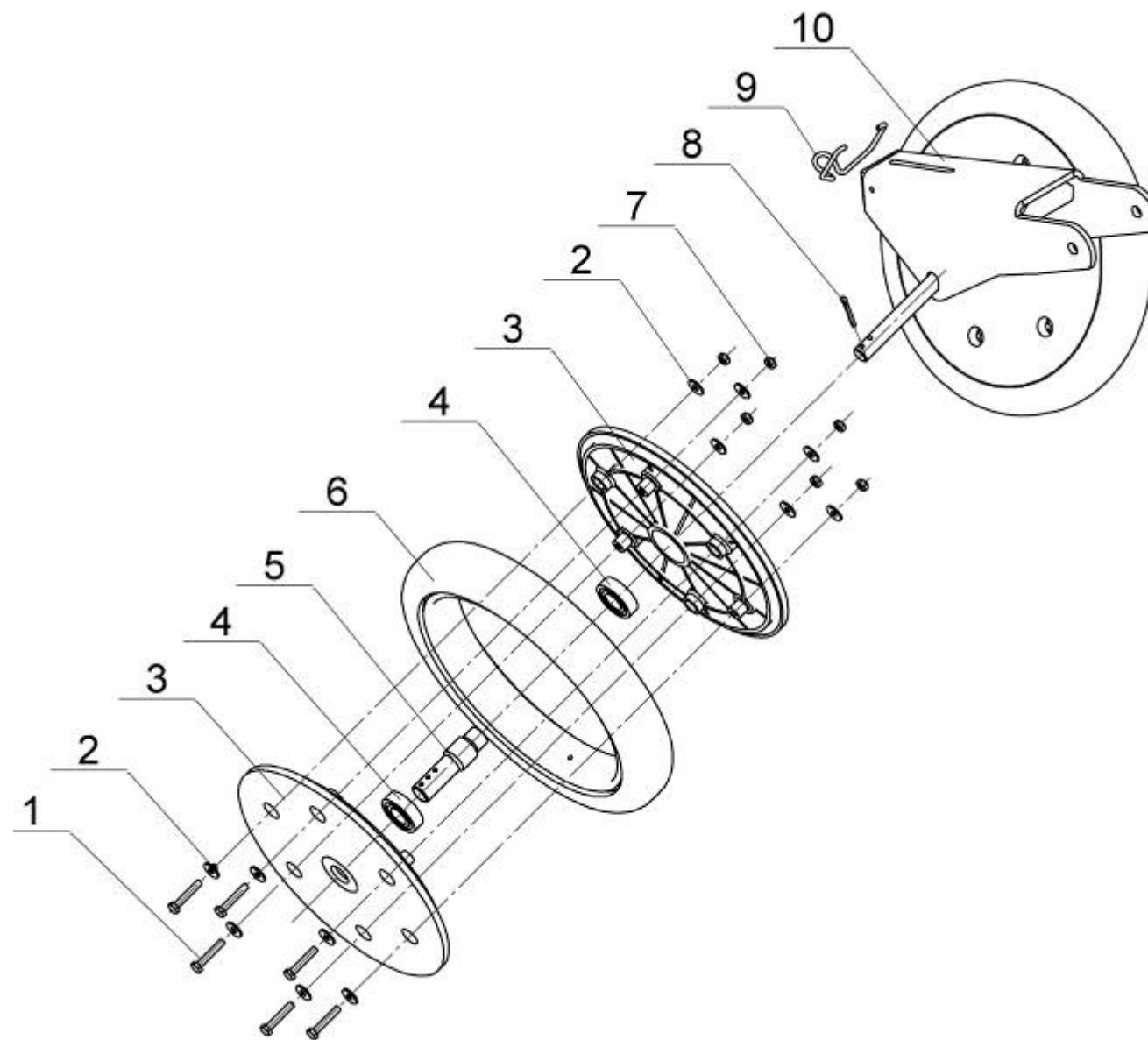
Рис.6- Каток прикатывающий СУС 00.260
