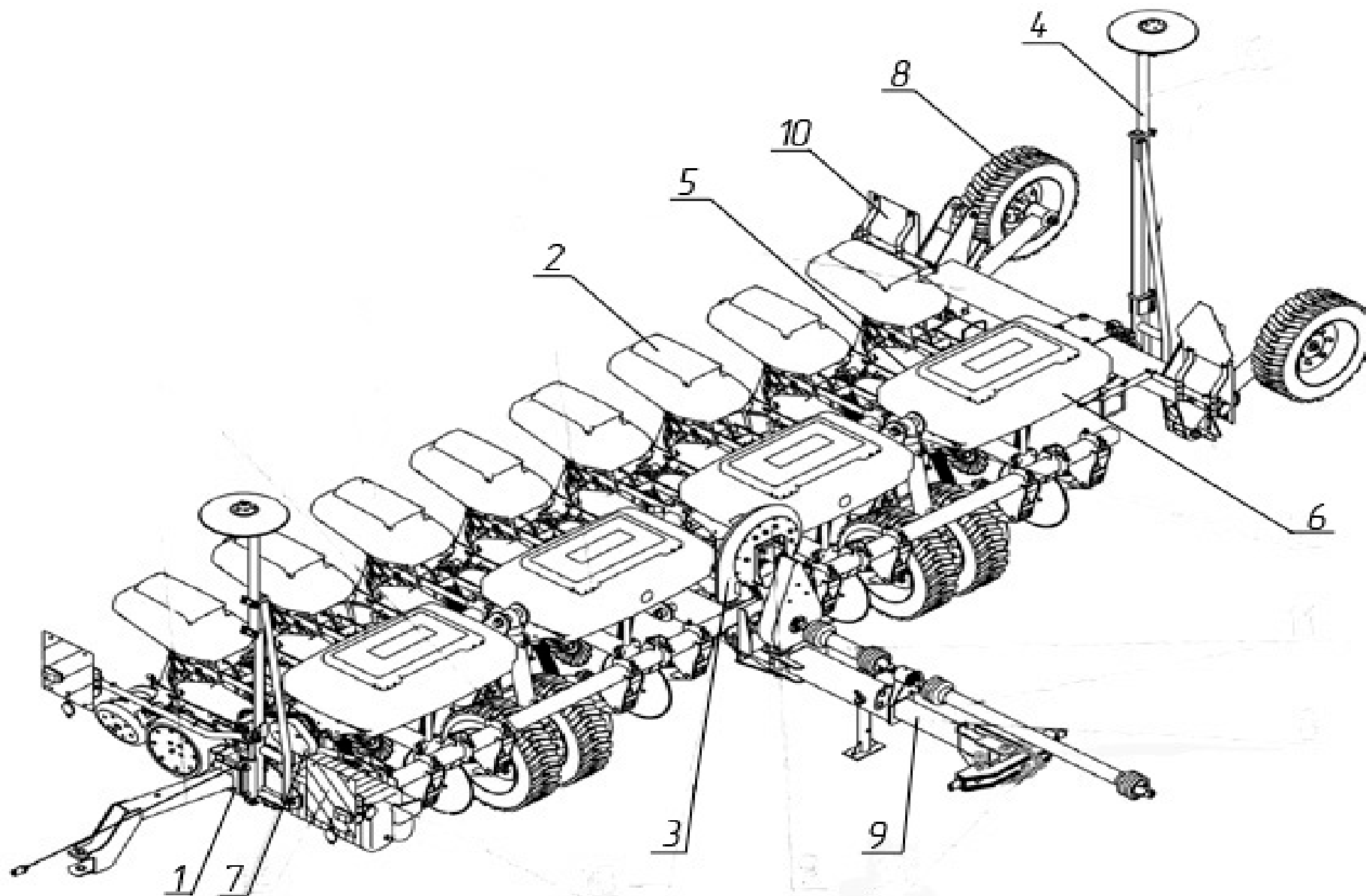
Рис. 2 Сеялка универсальная пневматическая Вега-8.
