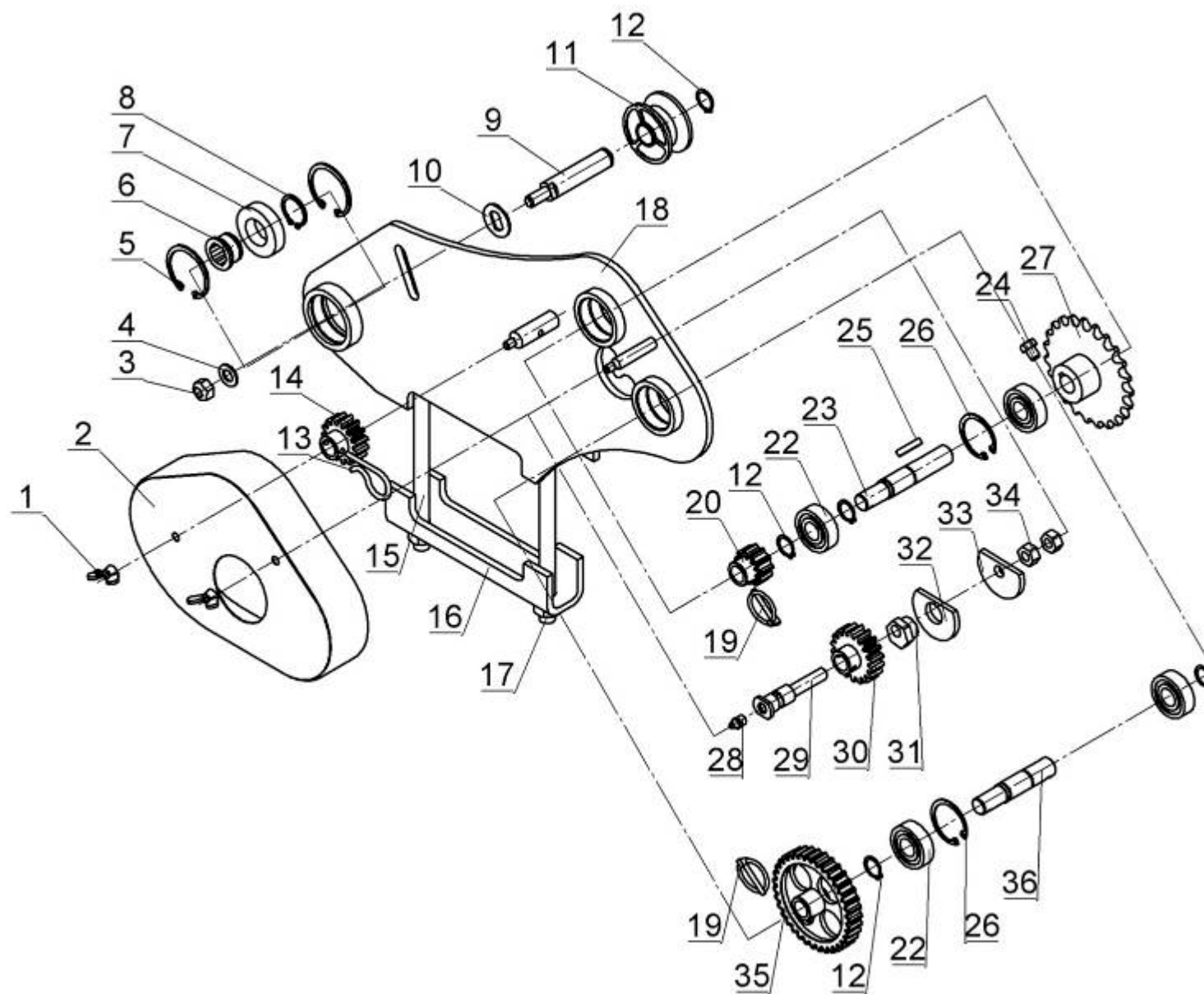
Рис.17- Редуктор СУС 00.5570А (правый) СУС 00.5570А-01(левый)
