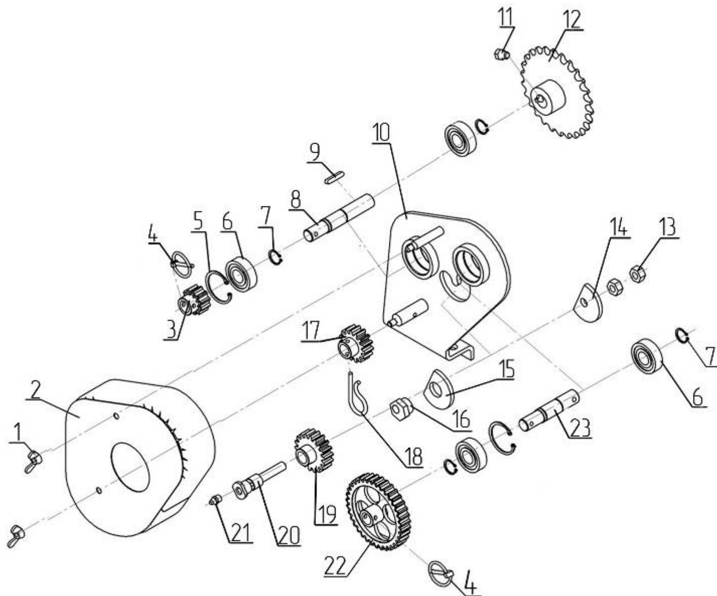
Рис.15 – Редуктор 509.046.5740А-02 (правый) Редуктор 509.046.5740А-03 (левый)
