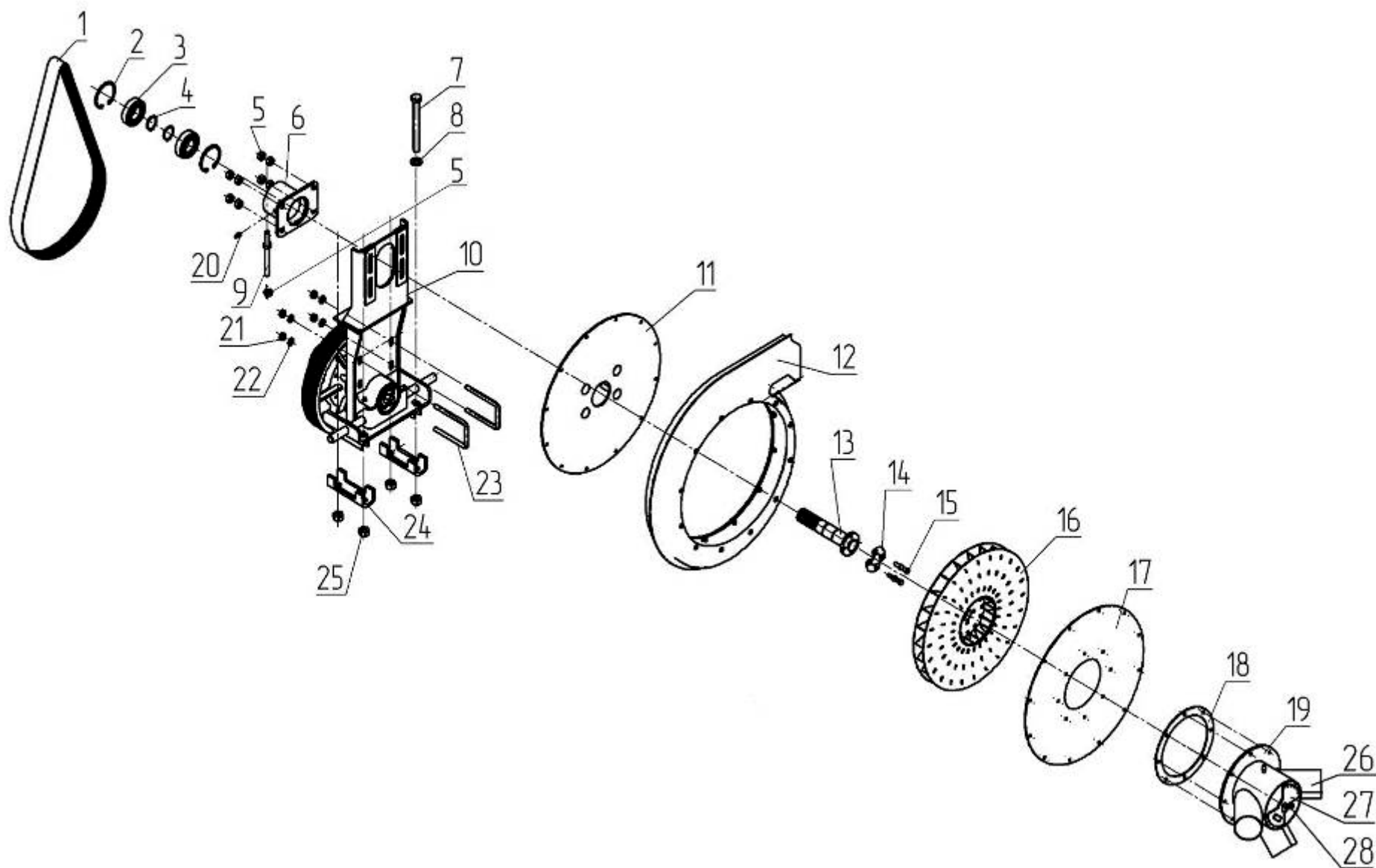
Рис.6 – Вентилятор 509.046.6150А (верхний вал)
