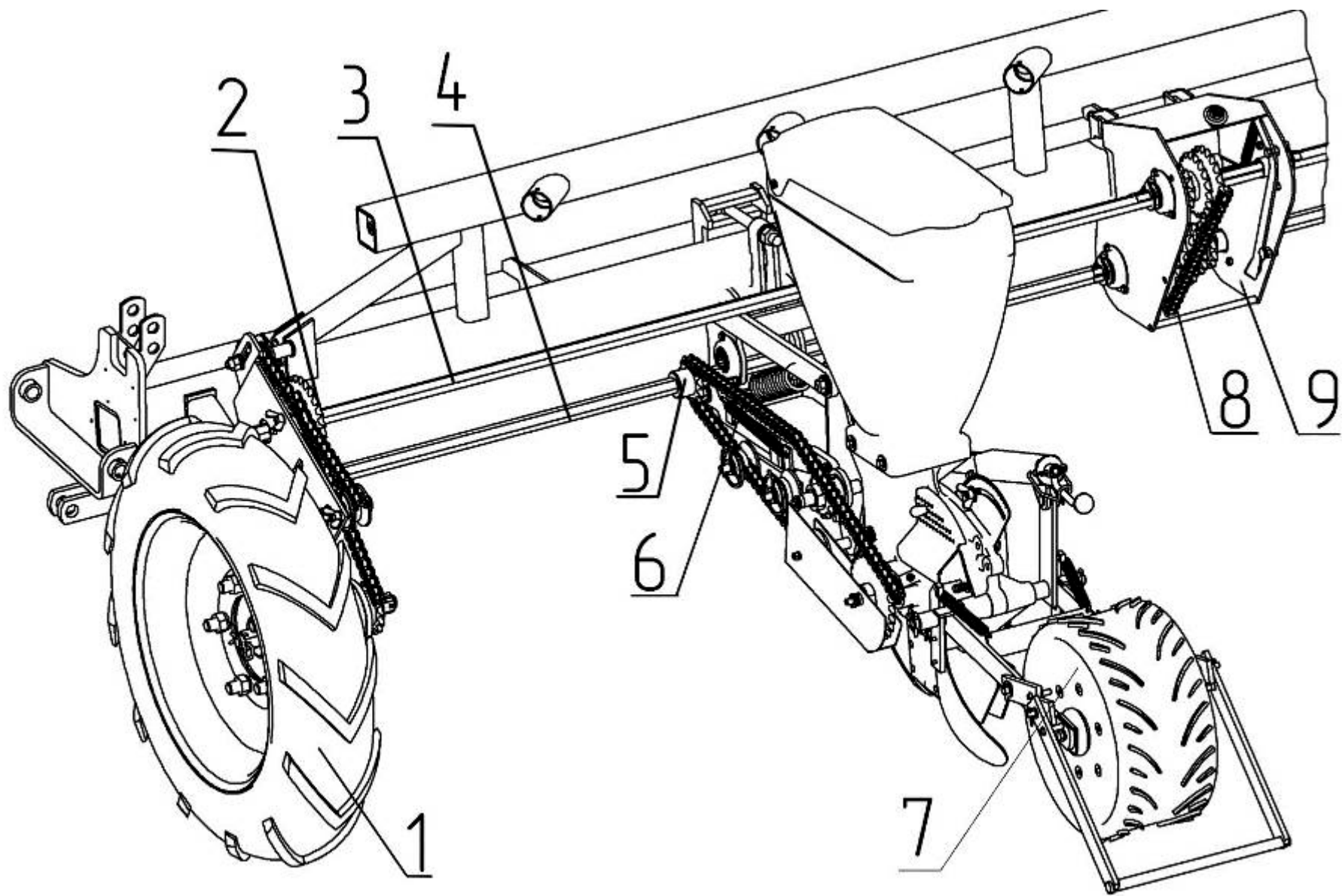
Рис.23 - Привод посевной секции 509.046.6100 до 01.08.2012 года одноконтурный привод
