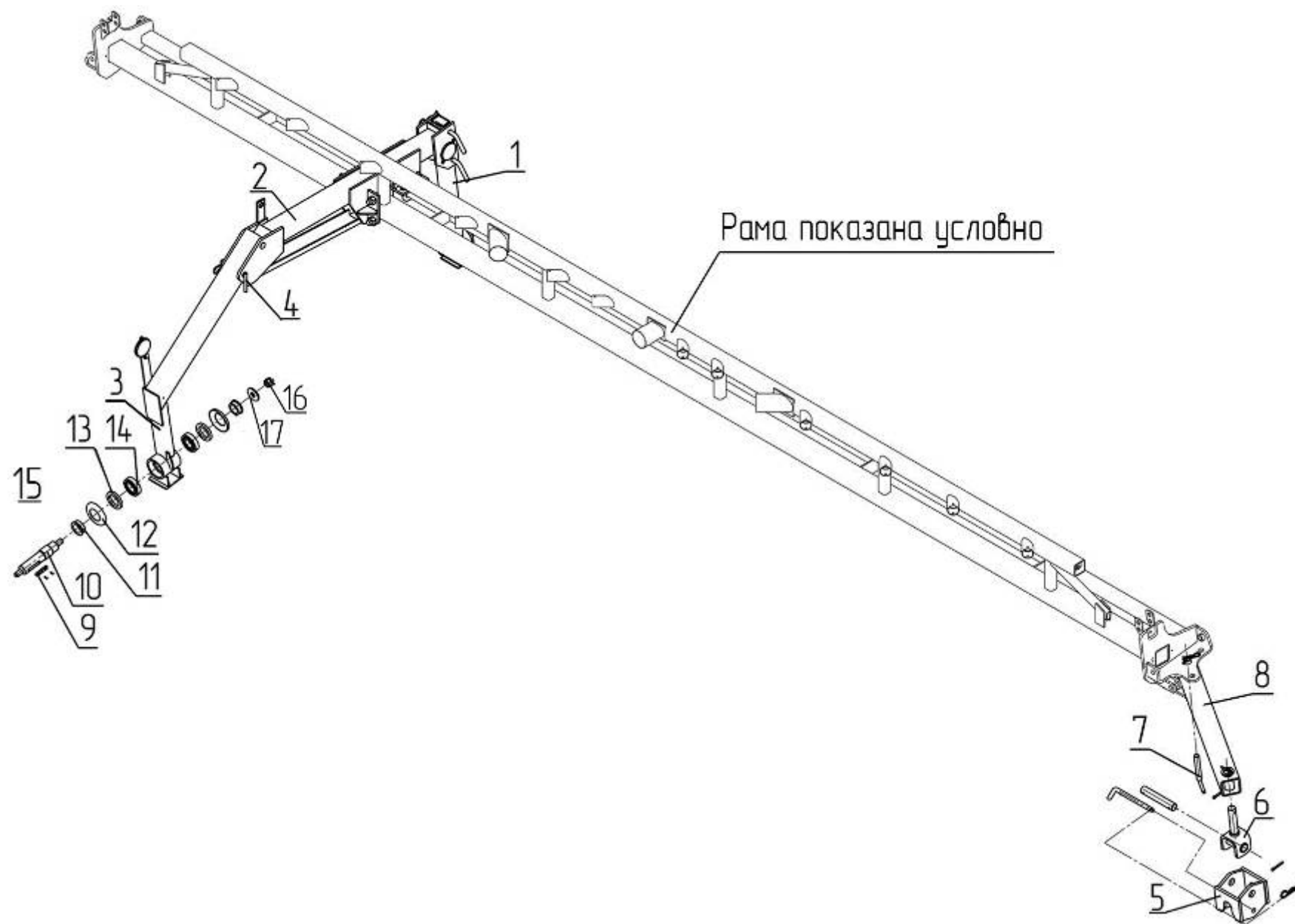
Рис.19 – Устройство транспортное 509.046.5820-01
