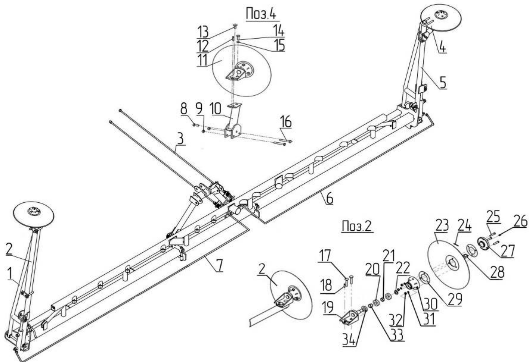
Рис.11 - Маркер 509.046.5610-01
