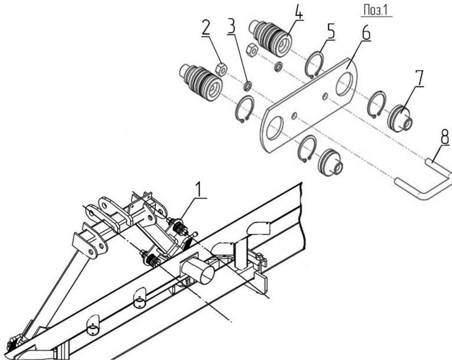
Рис.13 – Маркер 509.046.5610-01 Гидростыковочное устройство 509.046.6270
