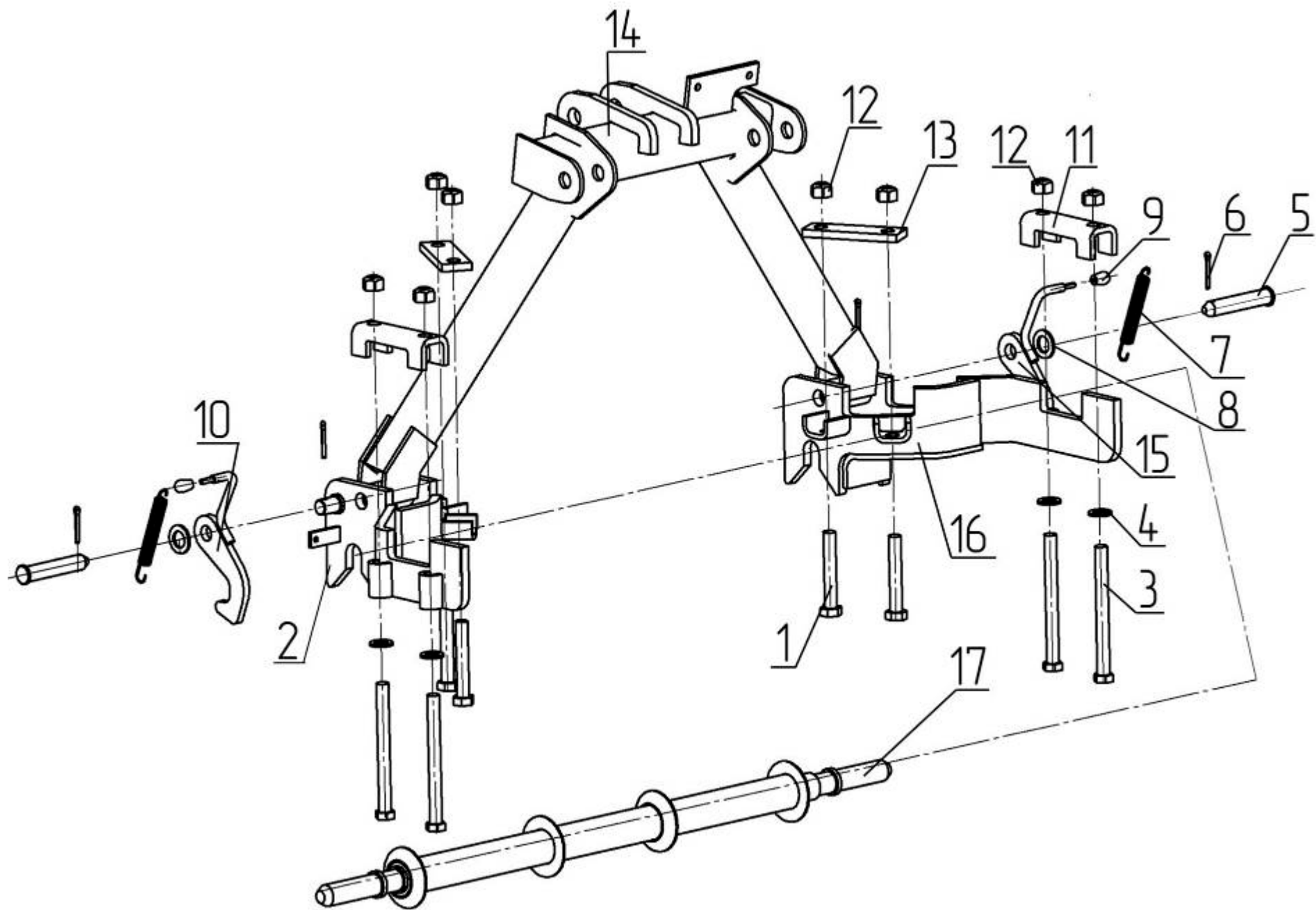
Рис.19 – Полуавтоматическая сцепка 509.046.6220
