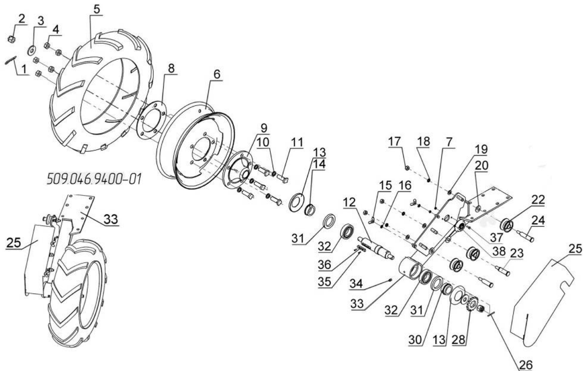
Рис.9 – Опорно-приводное колесо 509.046.9400 (левое) Опорно-приводное колесо 509.046.9400-01 (правое)
