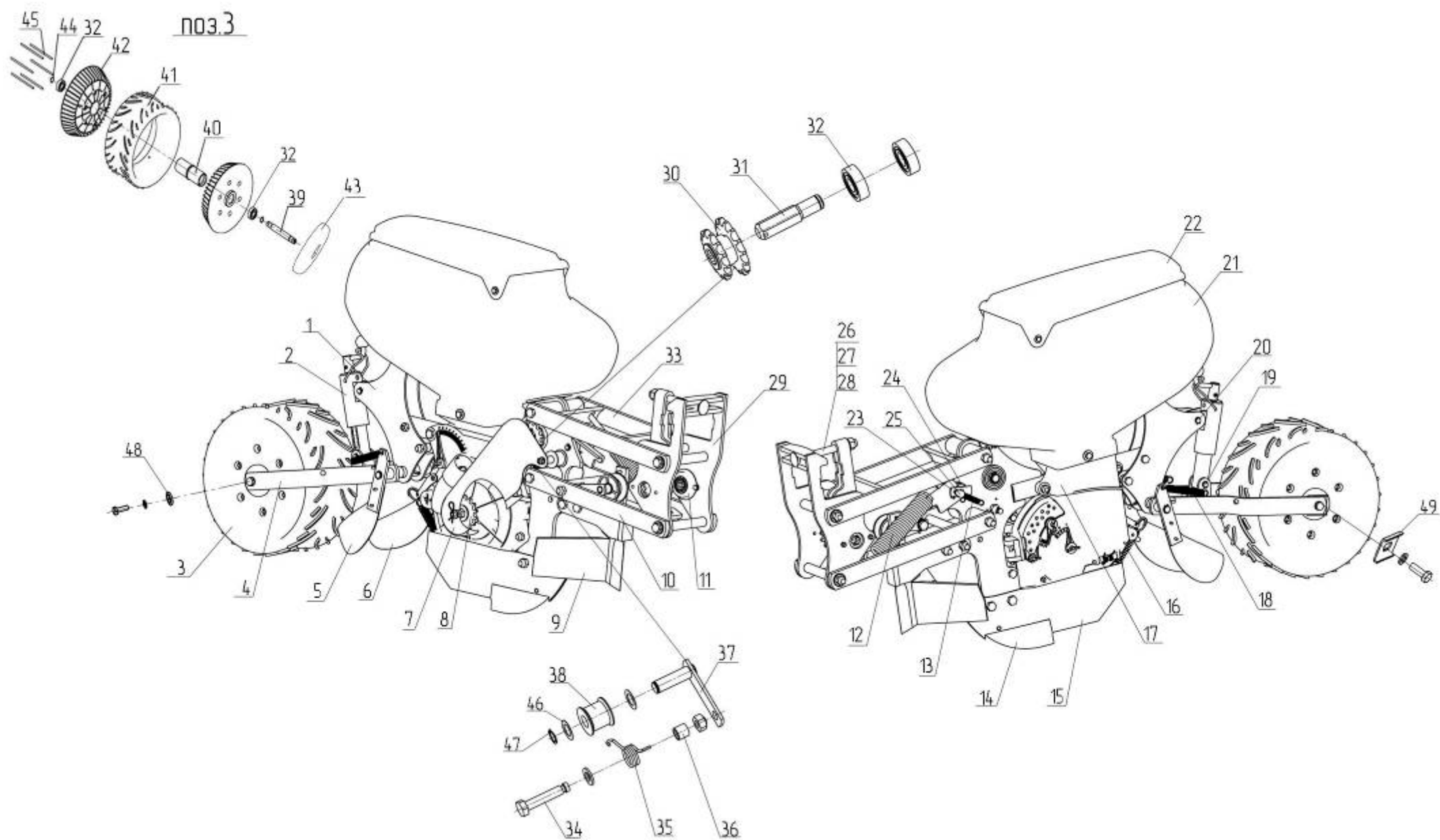
Рис.4 – Посевная секция 509.046.6800
