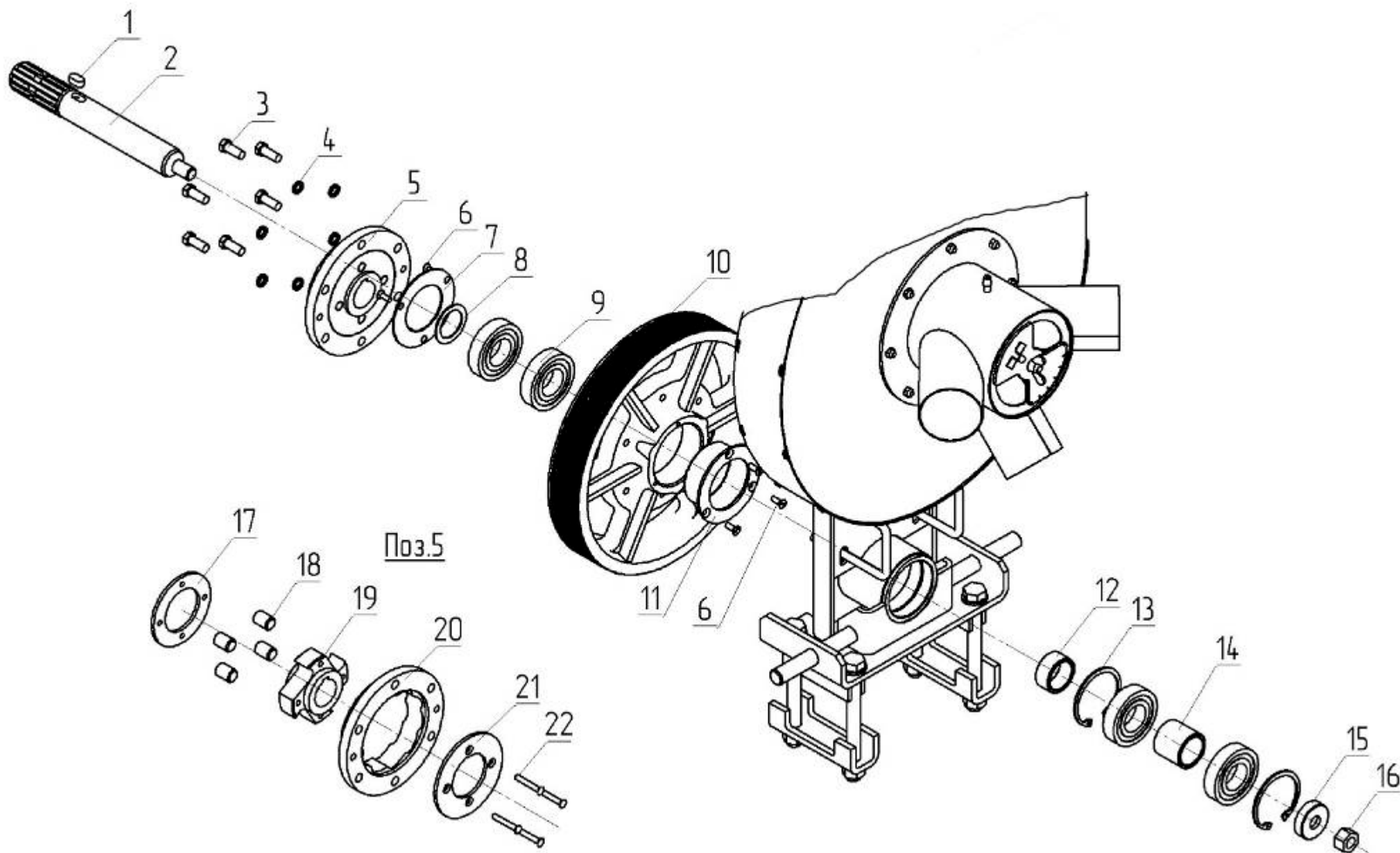
Рис.6 – Вентилятор 509.046.7710. Нижний вал
