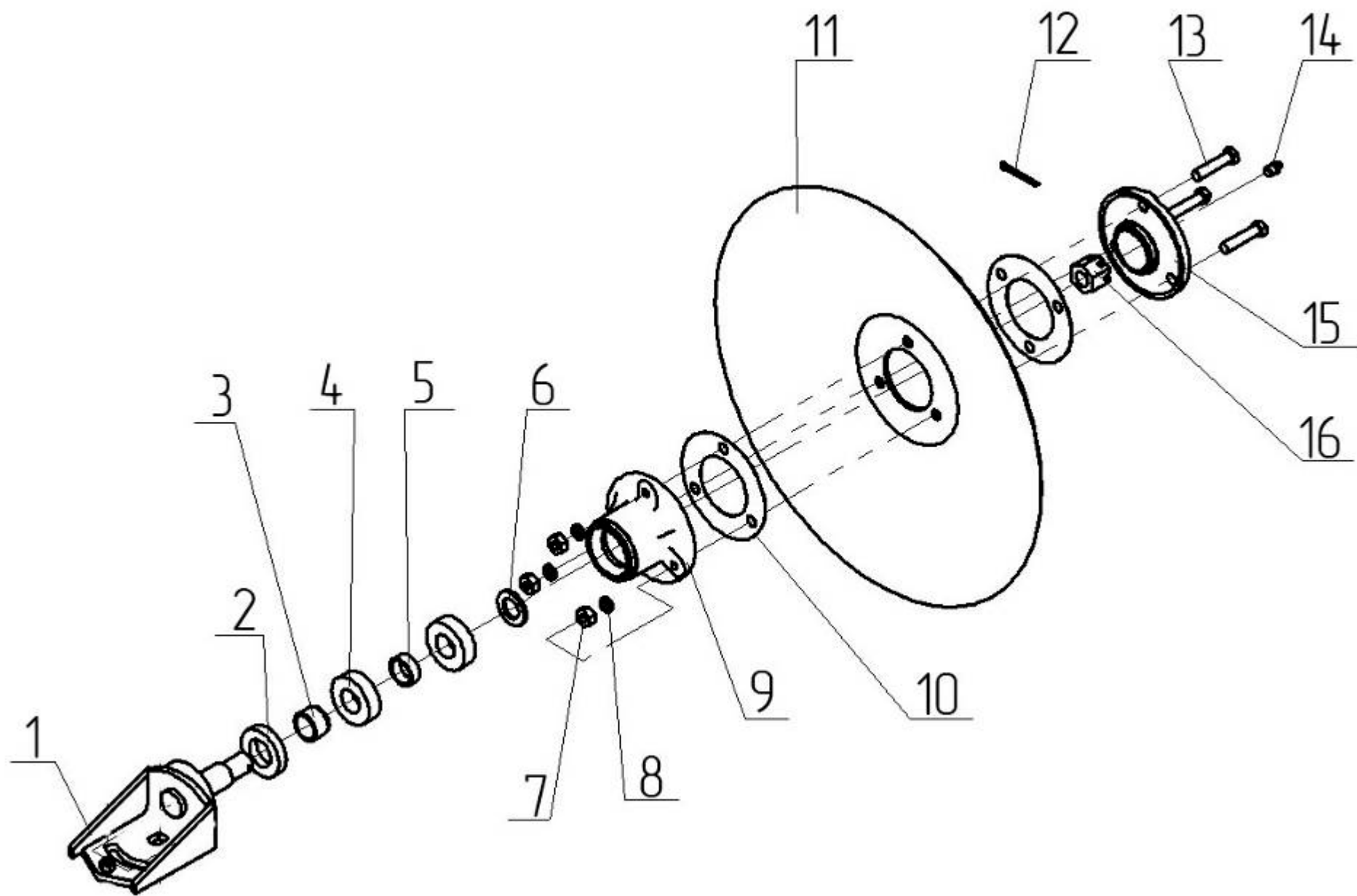
Рис.12 – Диск СШЕ 04.120
