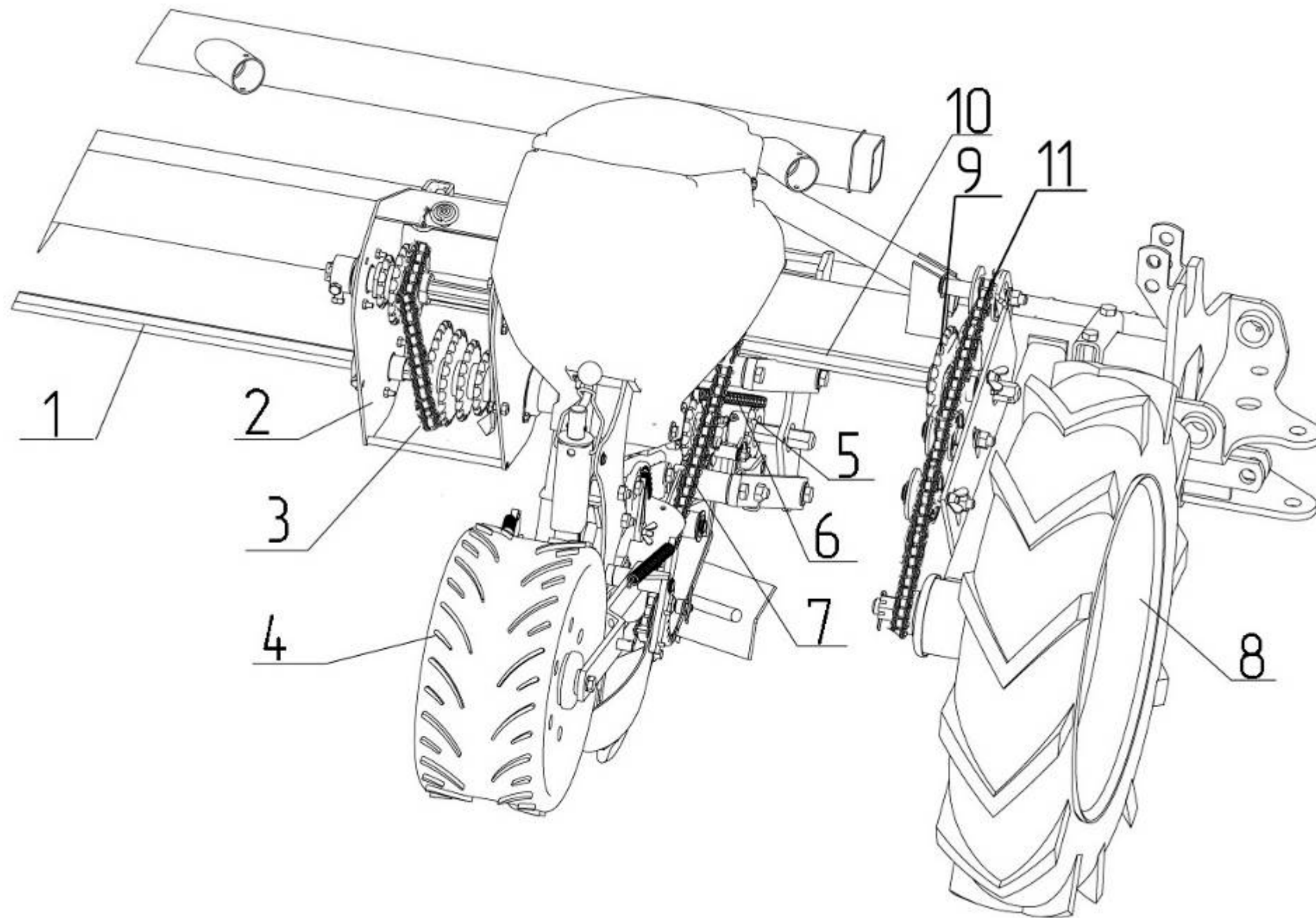
Рис.20 - Привод посевной секции 509.046.6800
