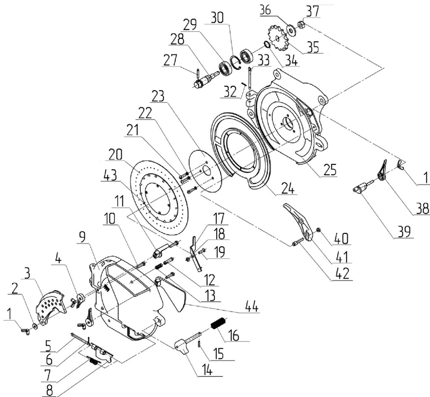
Рис.5 - Аппарат высевающий СУС 00.1400
