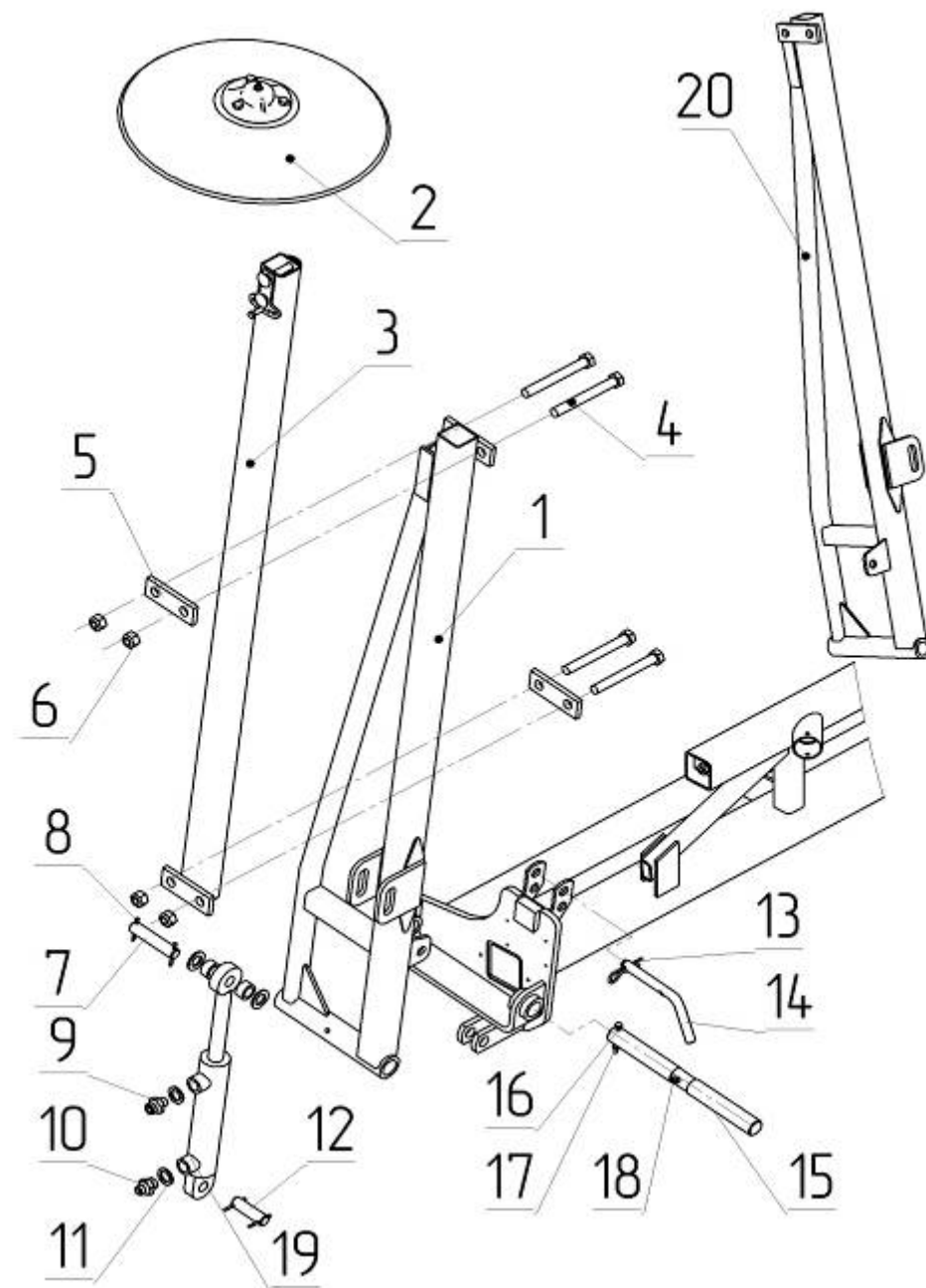
Рис.11 – Маркер. Штанга
