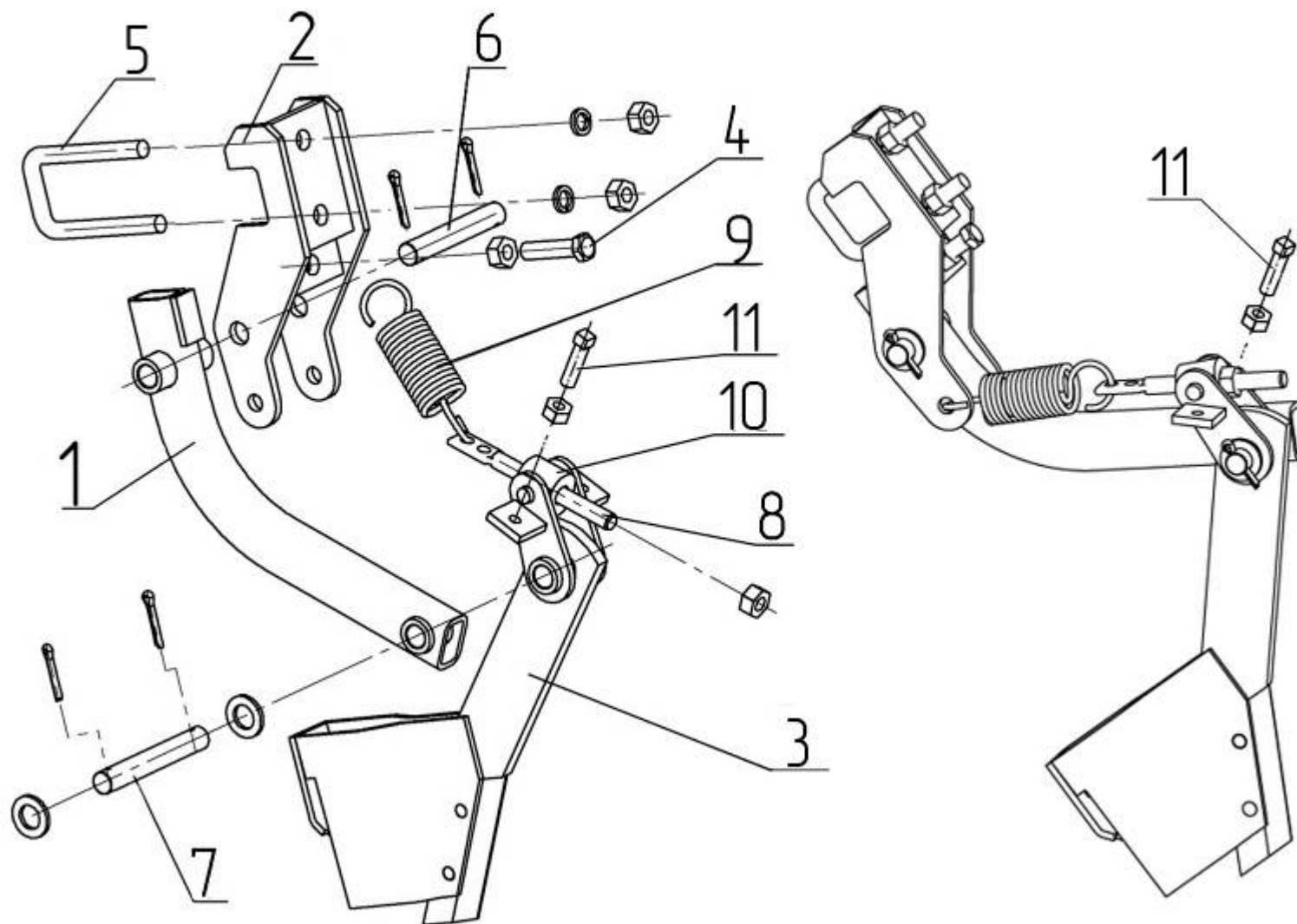
Рис.15 – Сошник туковый 509.046.2090 (правый) Сошник туковый 509.046.2090 -01 (левый)
