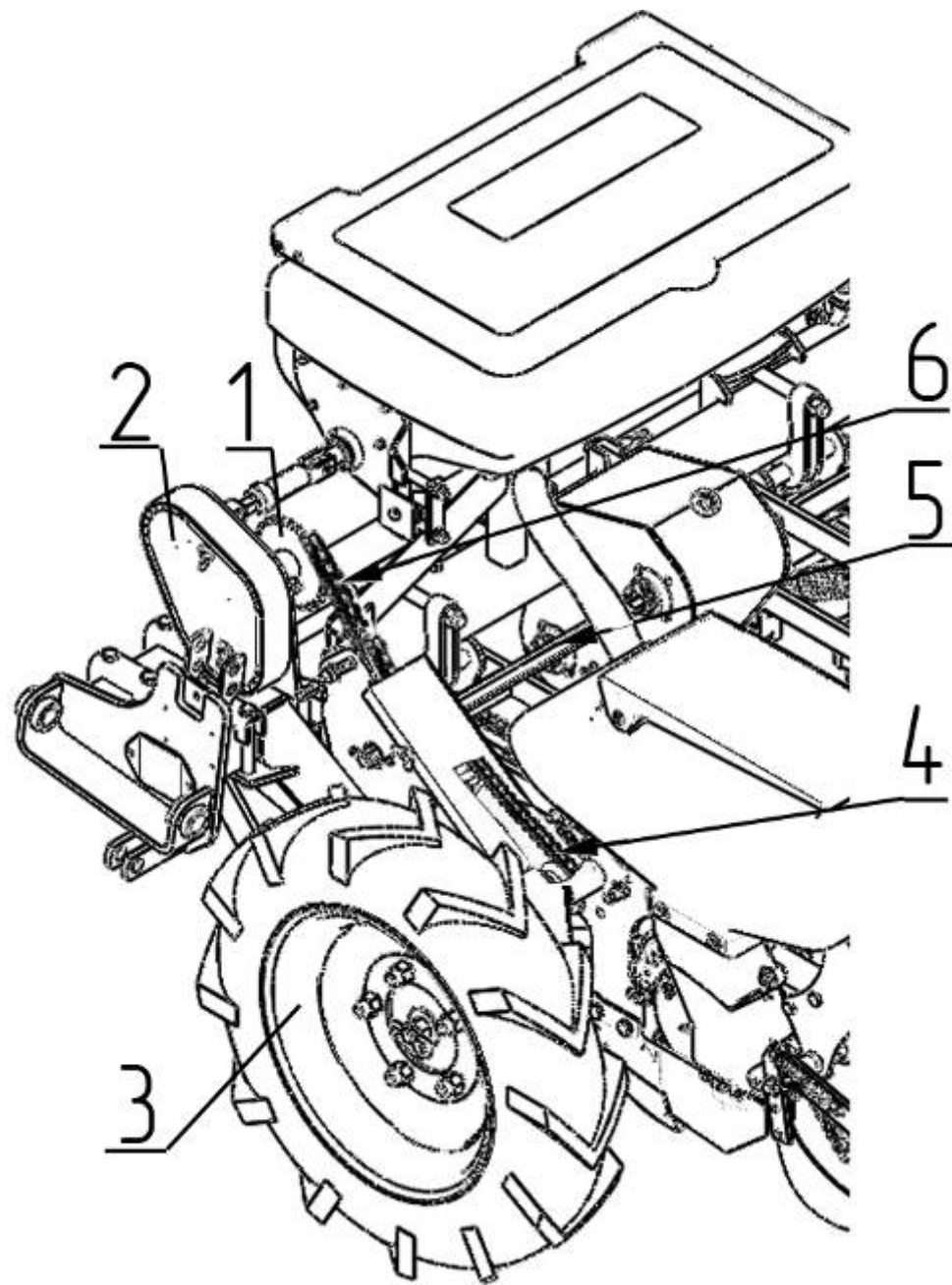
Рис.17 – Привод туковывевающего аппарата
