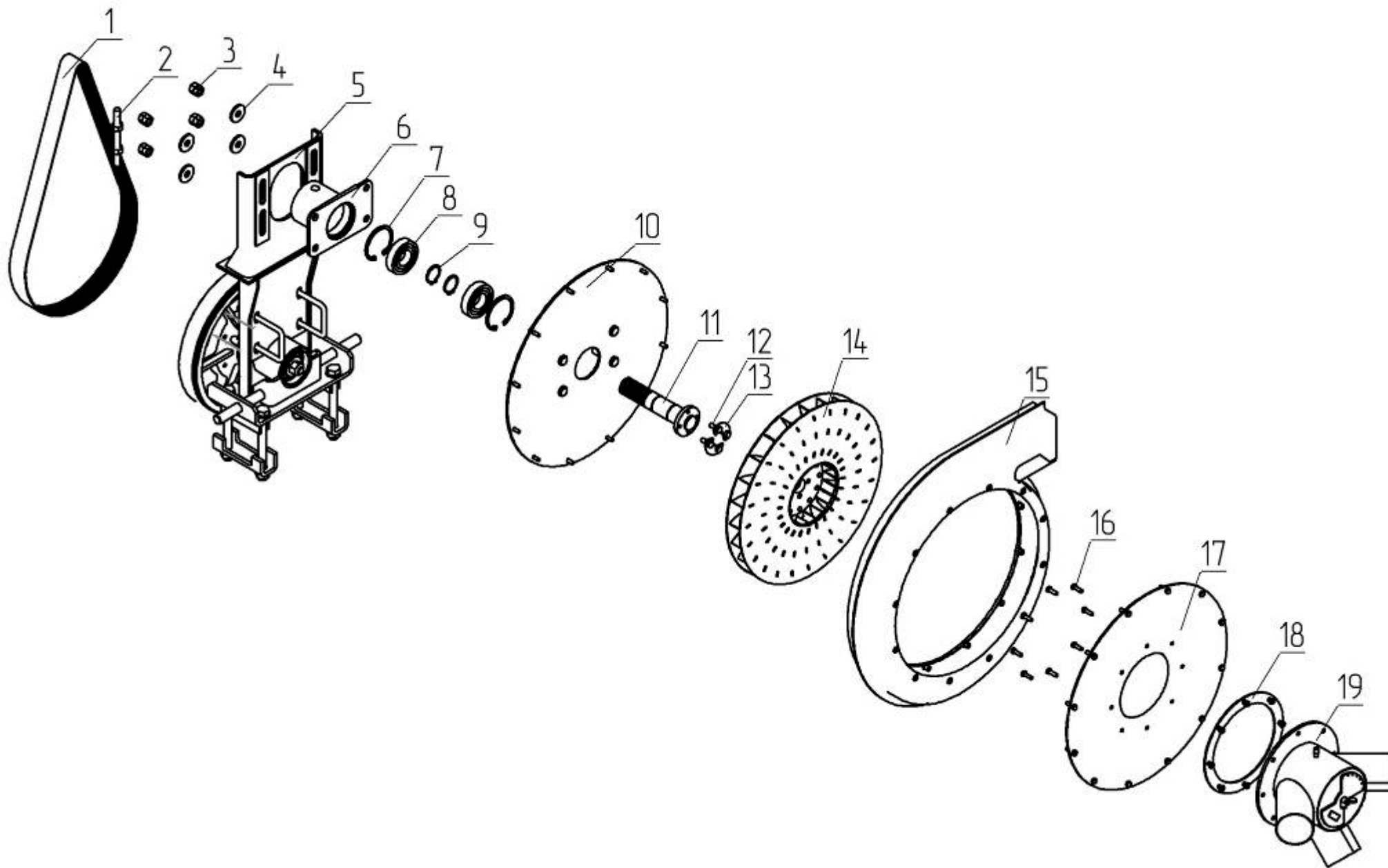
Рис.7 – Вентилятор 509.046.7710. Верхний вал
