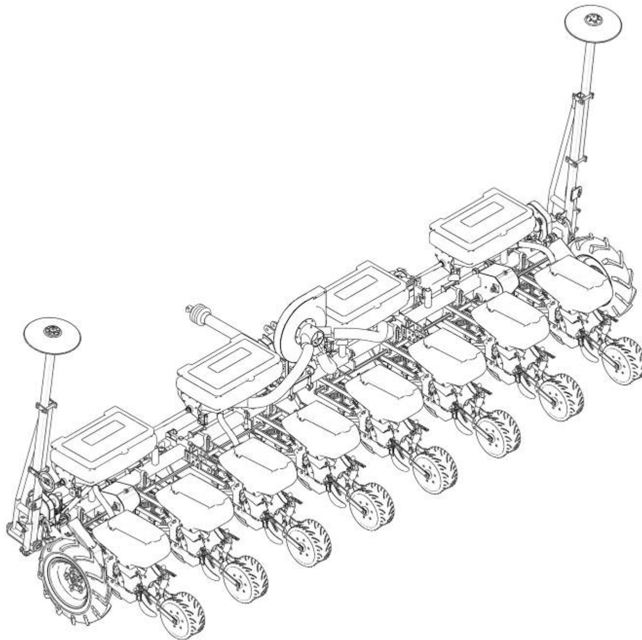
Рис. 3 – Сеялка универсальная пневматическая VESTA 6 PROFi (УПС-6А-02)
