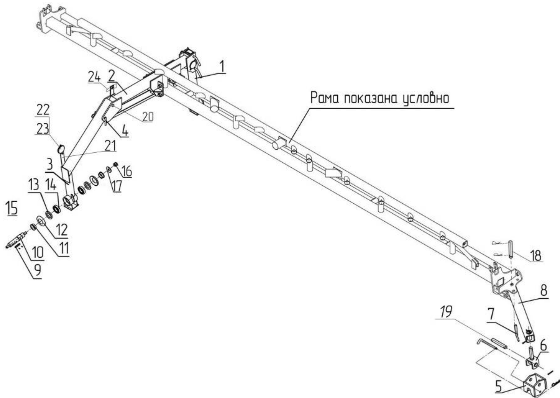
Рис.18 – Устройство транспортное 509.046.5820-01
