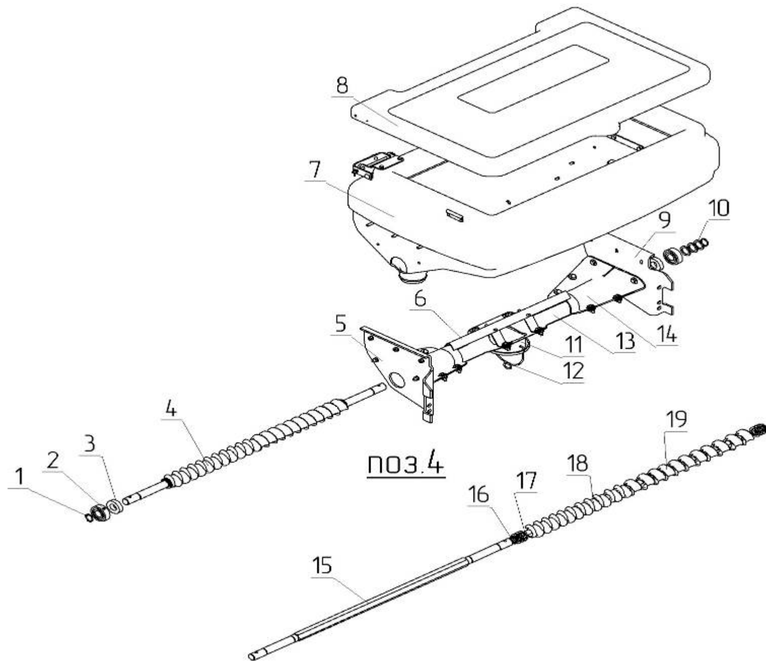
Рис.16 – Аппарат туковывсевающий 509.046.7870
