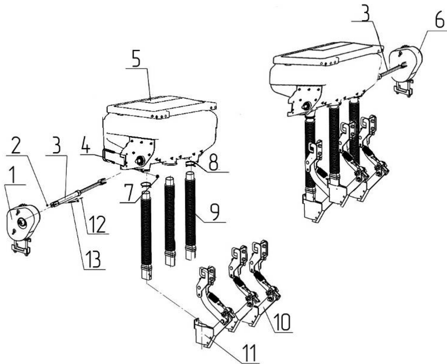
Рис.13 – Туковысевающая система сеялок «VESTA 6 PROFi» (УПС-6А; УПС-6А-02)
