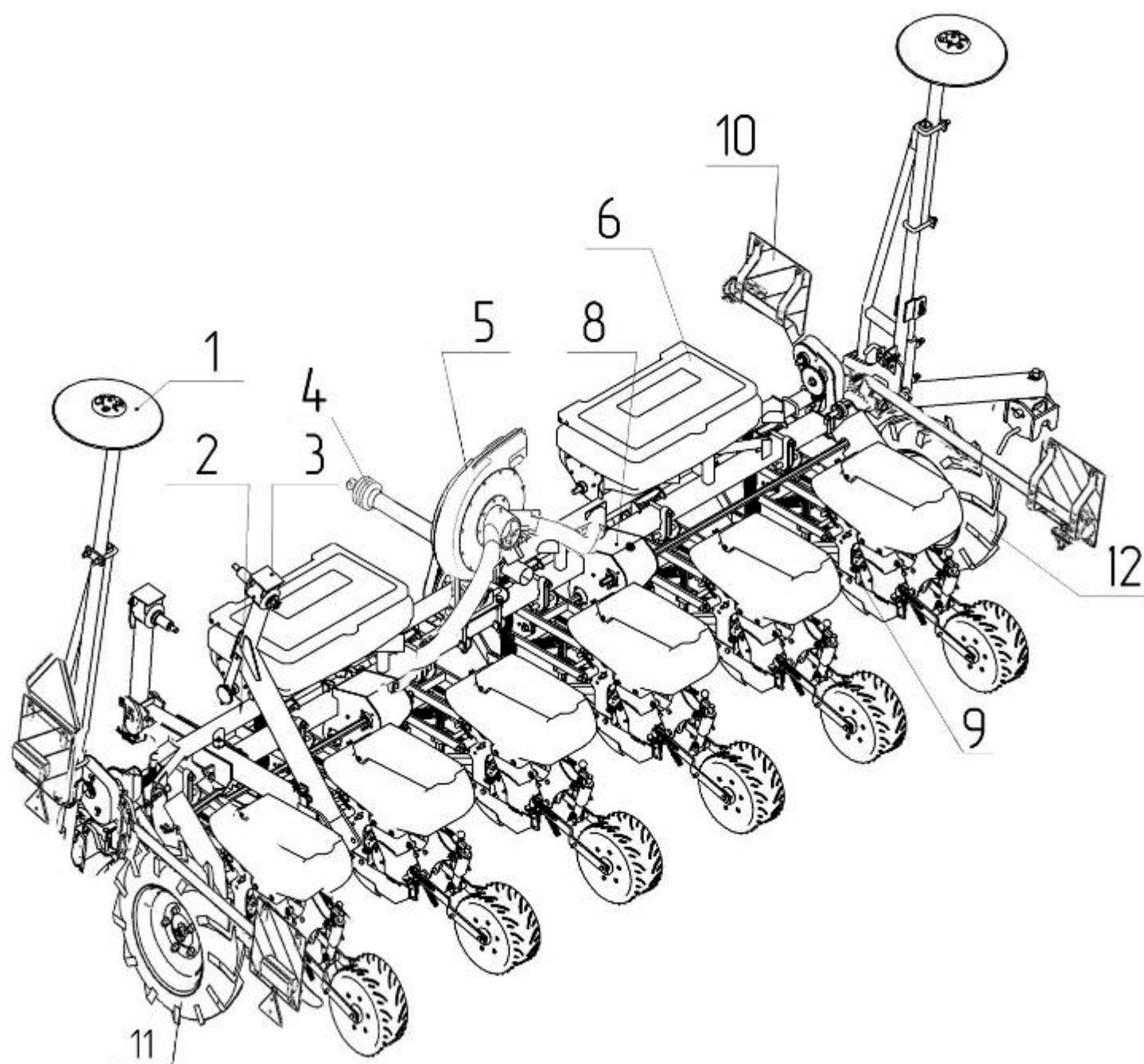
Рис. 1 – Сеялка универсальная пневматическая VESTA 6 PROFi (УПС-6А)
