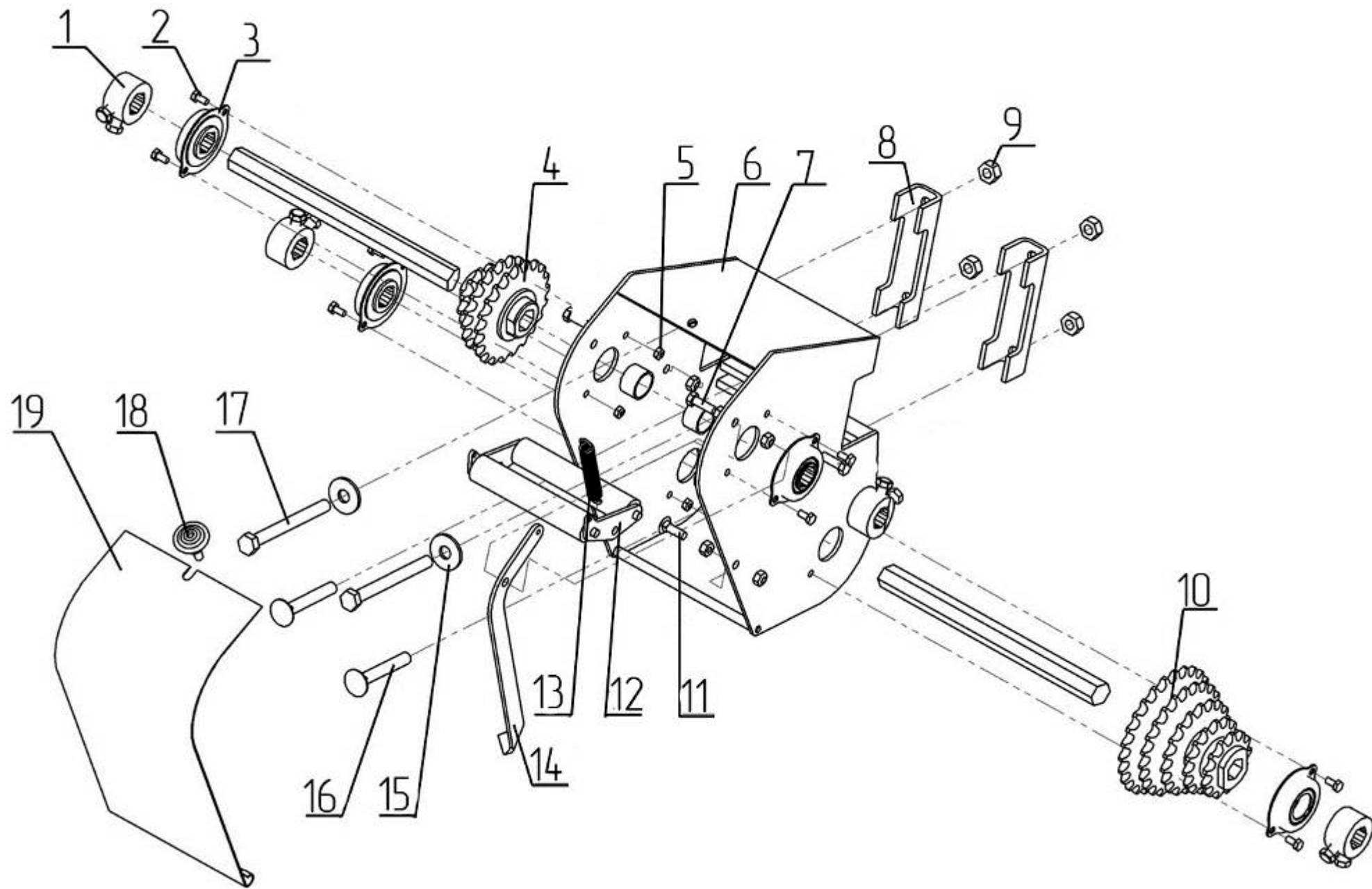
Рис.8 – Механизм передач 509.046.6060
