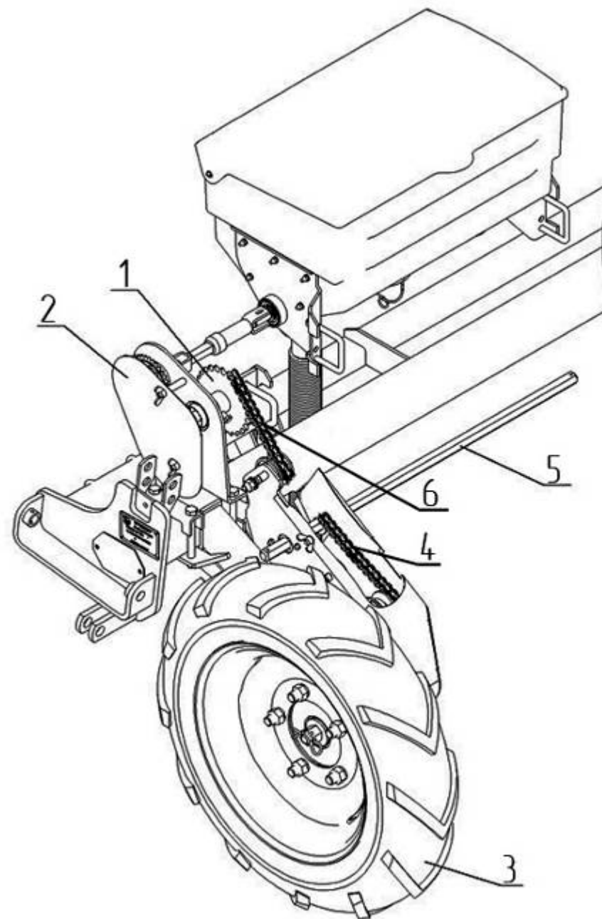
Рис.19 – Привод туковывсевающего аппарата
